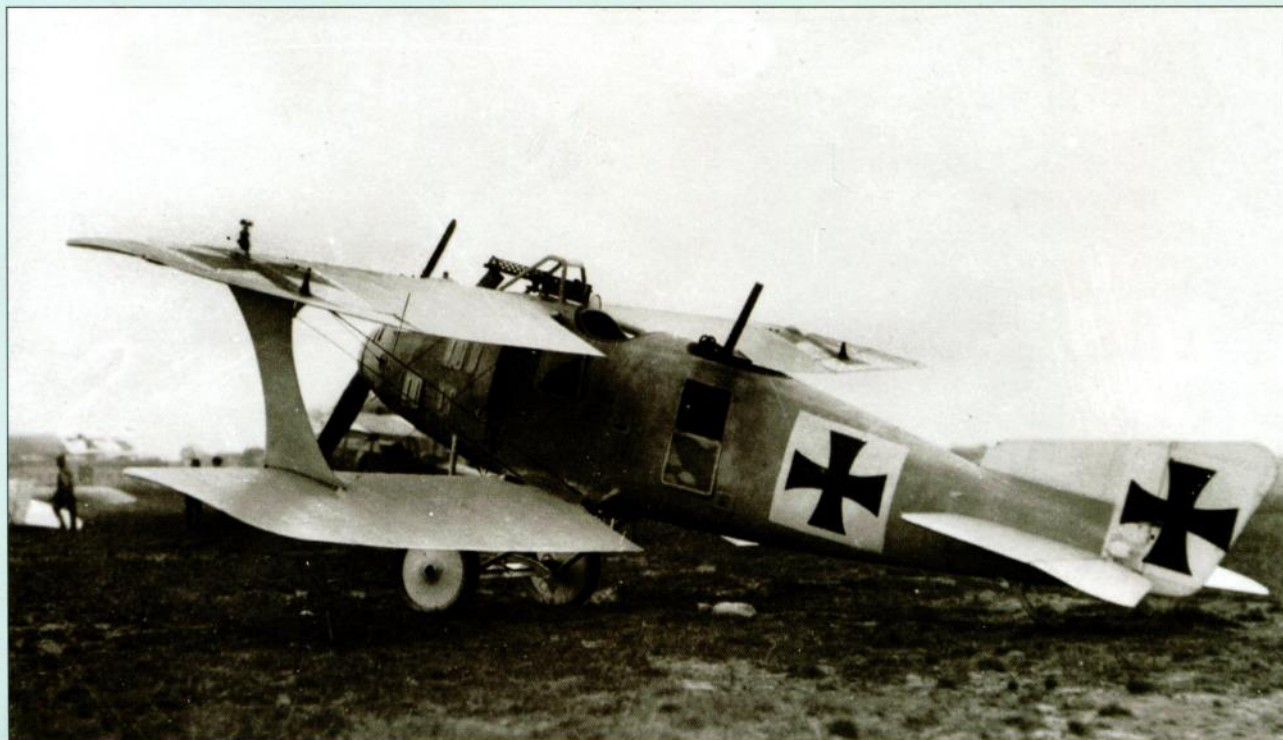
«Роланд» С.ИИ отличался монококовым фюзеляжем чистых аэродинамических форм
