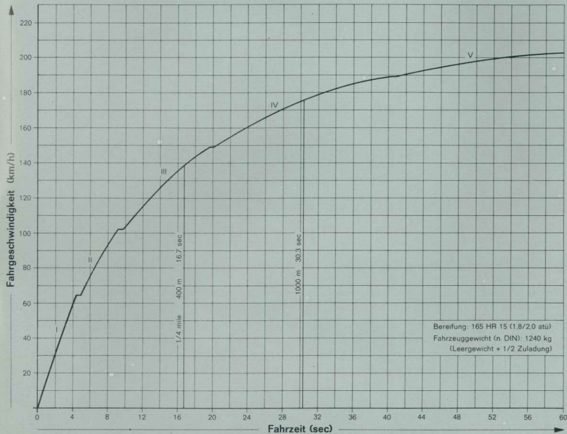
Beschleunigungsdiagramm Typ 911/2000
