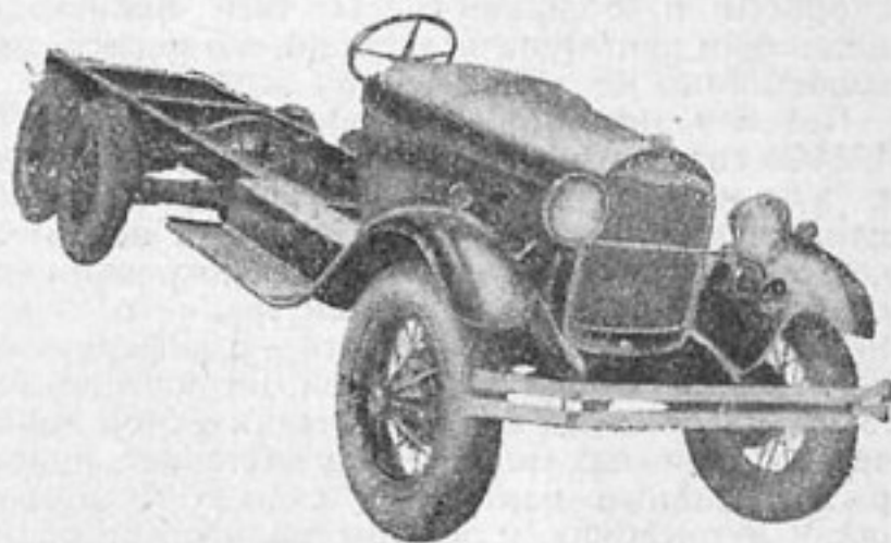
Шасси „Форда“ с третьей осью „Лонгфрам“
