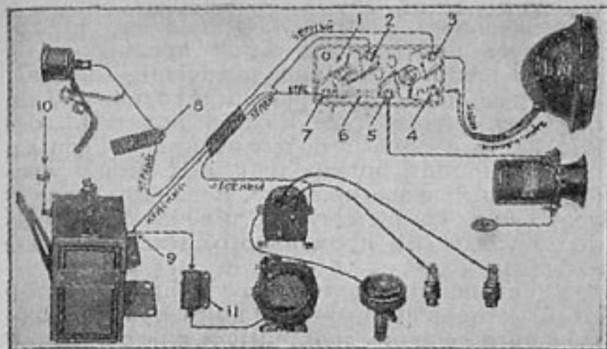
Фиг. 5. Схема електрооборудования мотоцикла „Харлей-Давидсон“ 1926—29 п.
