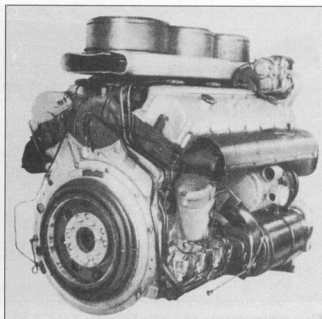
Двигатель HL230P45
