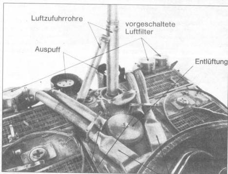
Крепление оборудования для подводного вождения на корме танка
