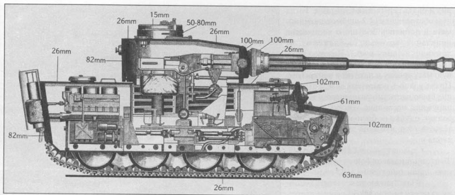
Схема бронирования танка «Тигр»
