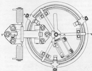
Люк механика-водителя
