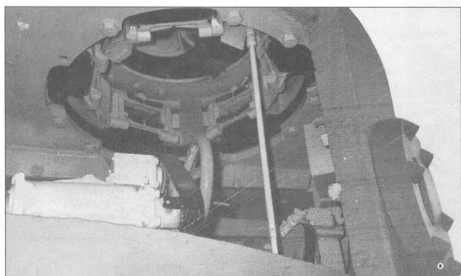
Командирская башенка «Тигров» ранних серий
