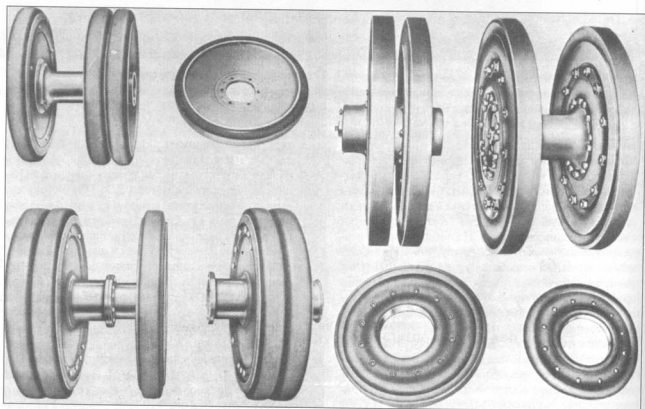
Опорные катки танка «Тигр». Слева - с резиновым бандажем машин ранних и средних выпусков, справа - без бандажа с внутренней амортизацией танков поздних серий.
