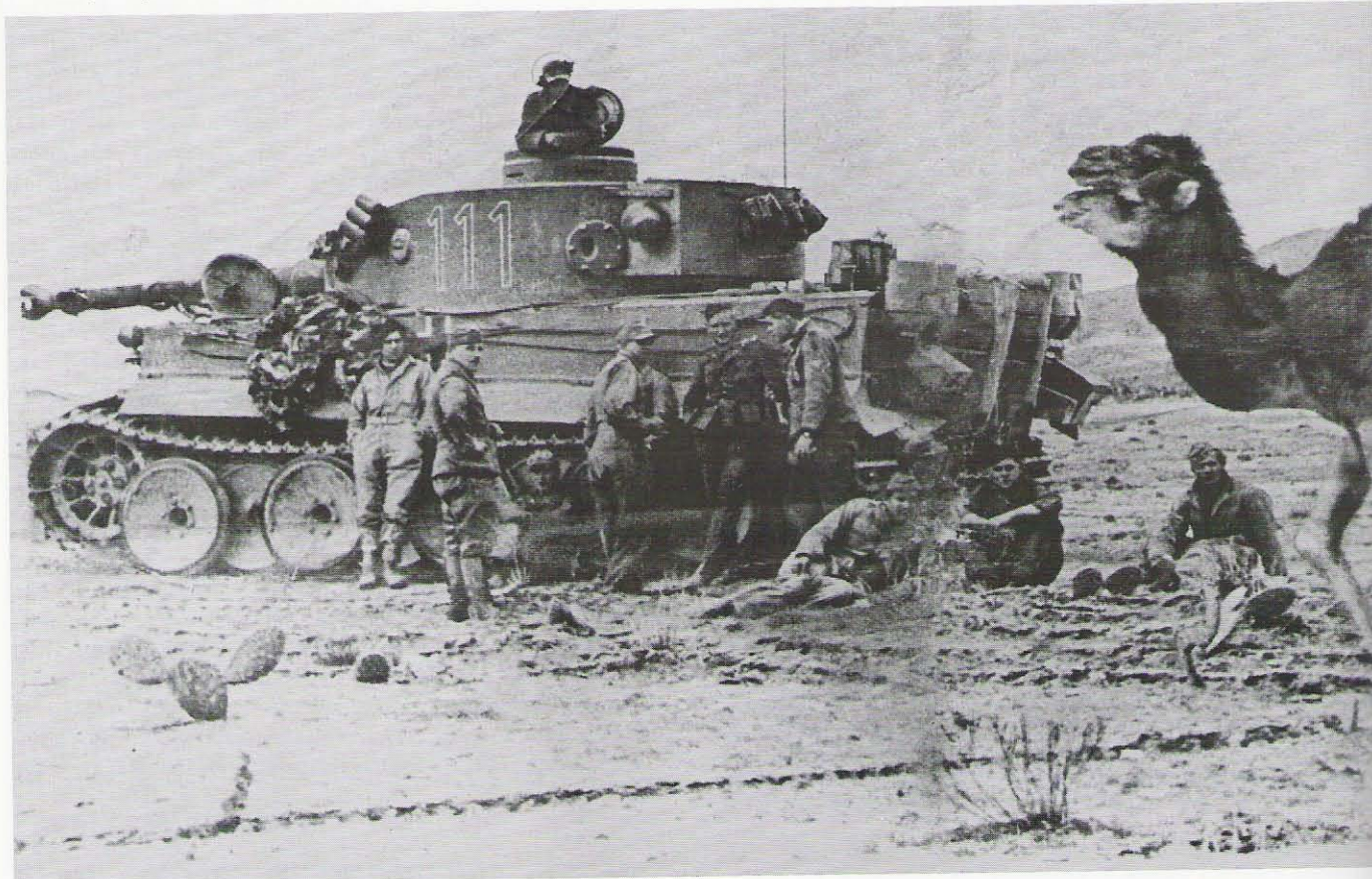
PzKpfw VI „Tiger” Ausf. H1 nr „111” z 1. kompanii 501. Batalionu Czołgów Ciężkich, Tunezja, grudzień 1942 roku. Z tyłu czołgu widoczne filtry typu Feifel. PzKpfw VI „Tiger” Ausf. H1 coded „111” tank of the 1st Company 501st schwere Heeres Panzer Abteilung , Tunisia, December 1942. Tank was equipped with Feifel-type air filters. [Tank Museum 379/A5]
