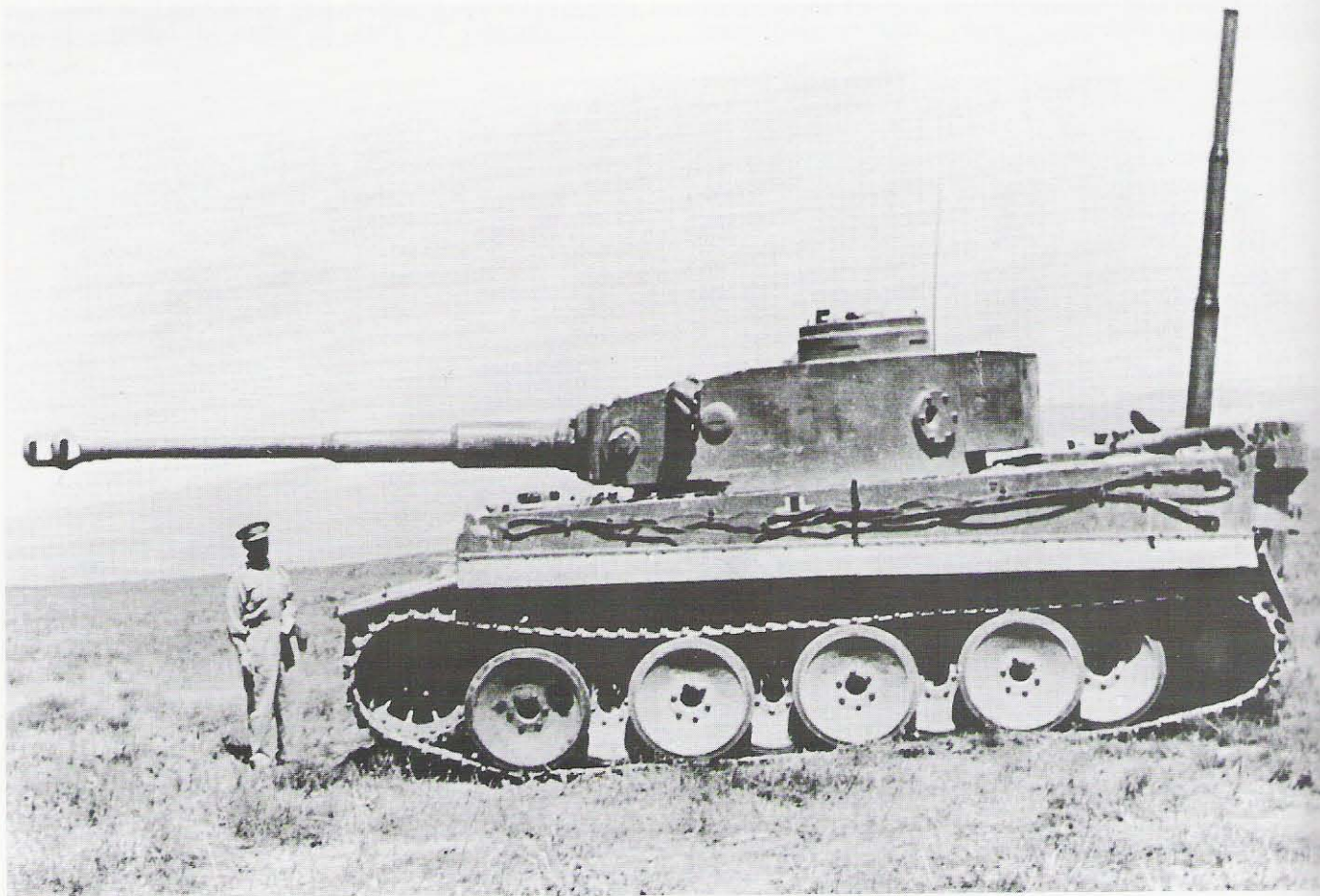
PzKpfw VI „Tiger” Ausf. H1 nr „131” z 1. kompanii 504. Batalionu Czołgów Ciężkich, Tunezja, kwiecień 1943 roku. Czołg posiada zamontowane wyposażenie do pokonywania przeszkód morskich po dnie. PzKpfw VI “Tiger” Ausf. H1 coded No “131” tank of 1st Company 504th schwere Heeres Panzer Abteilung, Tunisia, April 1943. Tank fitted with deep wading equipment. [Tank Museum 291/C4]
