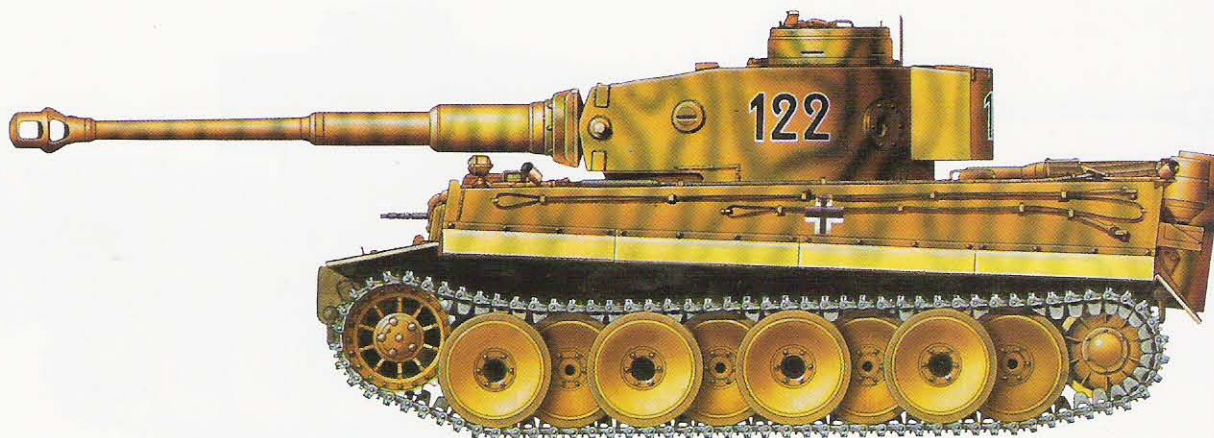
PzKpfw VI Sd Kfz 181 Ausf. H1 „Tiger“ z 1. kompanii 503. Batalionu Czołgów Ciężkich, Kursk, lipiec 1943 roku. PzKpfw VI Sd Kfz 181 Ausf. H1 “Tiger” of the 1st Company 503rd schwere Heeres Panzer Abteilung, Kursk, July 1943.
