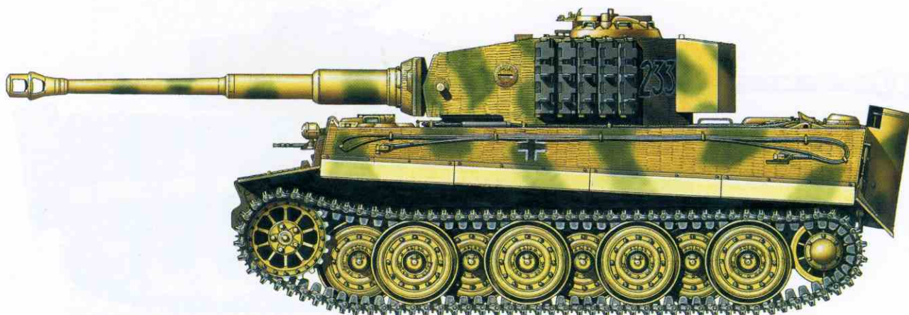
PzKpfw VI Sd Kfz 181 Ausf. E „Tiger“ z 510. Batalionu Czołgów Ciężkich, Litwa, lipiec 1944 roku. PzKpfw VI Sd Kfz 181 Ausf. E “Tiger” of the 510th schwere Heeres Panzer Abteilung, Lithuania, July 1944.
