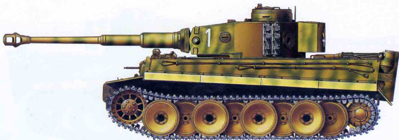
PzKpfw VI Sd Kfz 181 Ausf. E „Tiger“ z 1. kompanii 506. Batalionu Czołgów Ciężkich, front wschodni, wiosna 1944 roku. PzKpfw VI Sd Kfz 181 Ausf. E “Tiger” of the 1st Company 506th schwere Heeres Panzer Abteilung, Eastern Front, Spring 1944.
