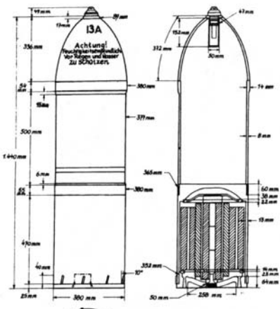
38 cm Raketen-Sprenggranate 4581
