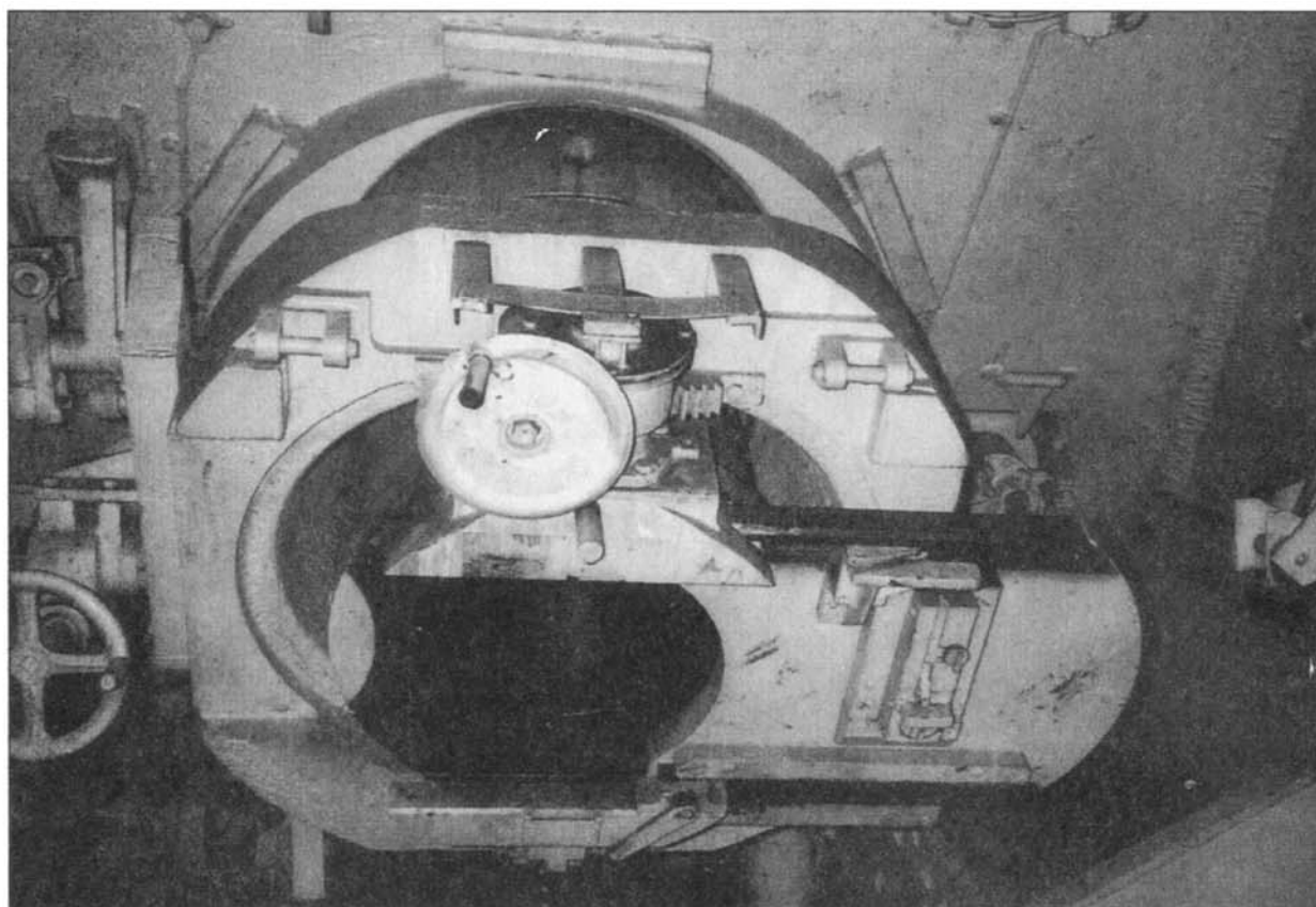
Казенная часть ракетомета RW 61
