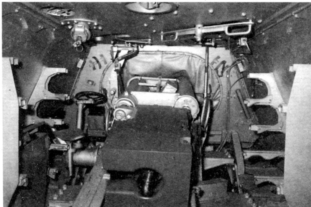
Боевое отделение САУ «Ягдтигр». На переднем плане — казенная часть 128-мм пушки. Слева от нее — рабочее место наводчика и маховик горизонтальной наводки. Над ним, в крыше рубки, установлено так называемое «устройство ближнего боя» — казнозарядная мортирка для стрельбы дымовыми и осколочными гранатами. По бортам рубки — стеллажи для пеналов с зарядами
