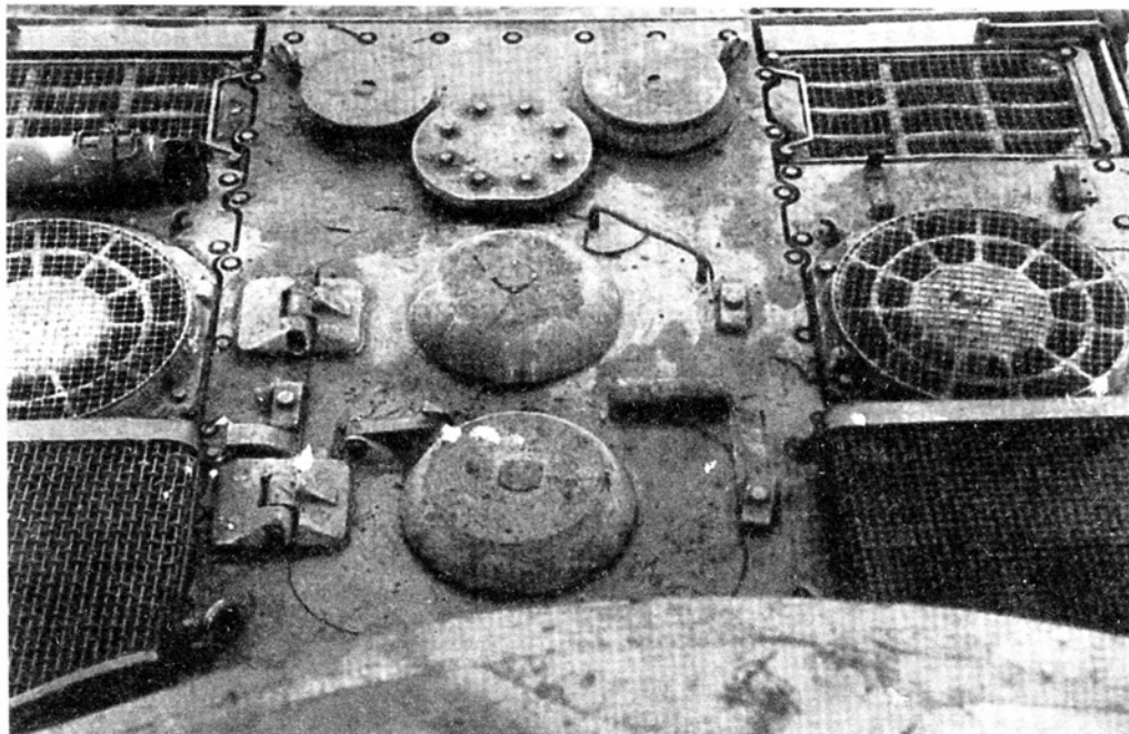
Вид на крышу моторного отделения. Прямоугольные литые решетки закрывают отверстия для притока воздуха, круглые — для его отвода. Заглушка в центре крыши установлена на отверстие для установки трубы ОПВТ
