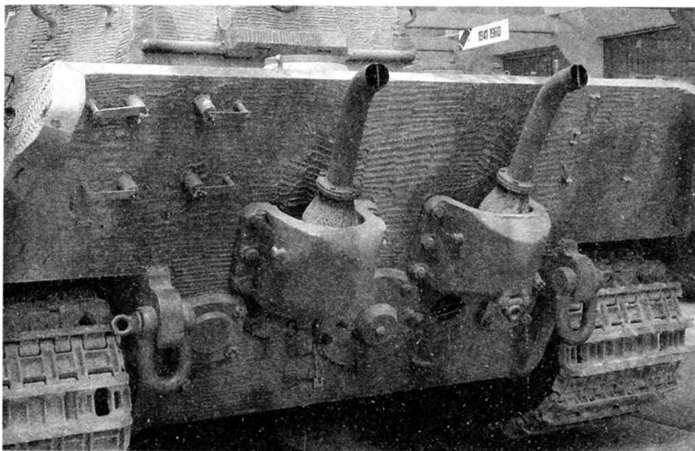
Кормовая часть корпуса. Под правой выхлопной трубой — не заглушенное отверстие для ручного запуска двигателя
