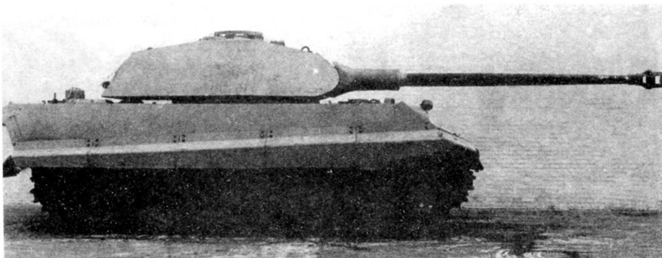
Первый прототип танка «Тигр II» (шасси V1) с башней «типа Порше» во дворе завода
