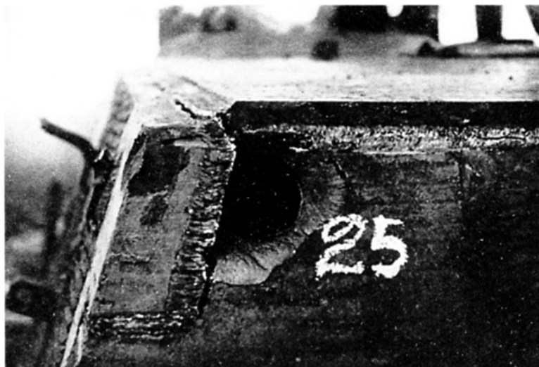
Лобовая и кормовая части башни танка № 102 после испытаний обстрелом. Пробоины 25 сделаны с дистанции 400 м 88-мм снарядом, прошедшим навывлет
