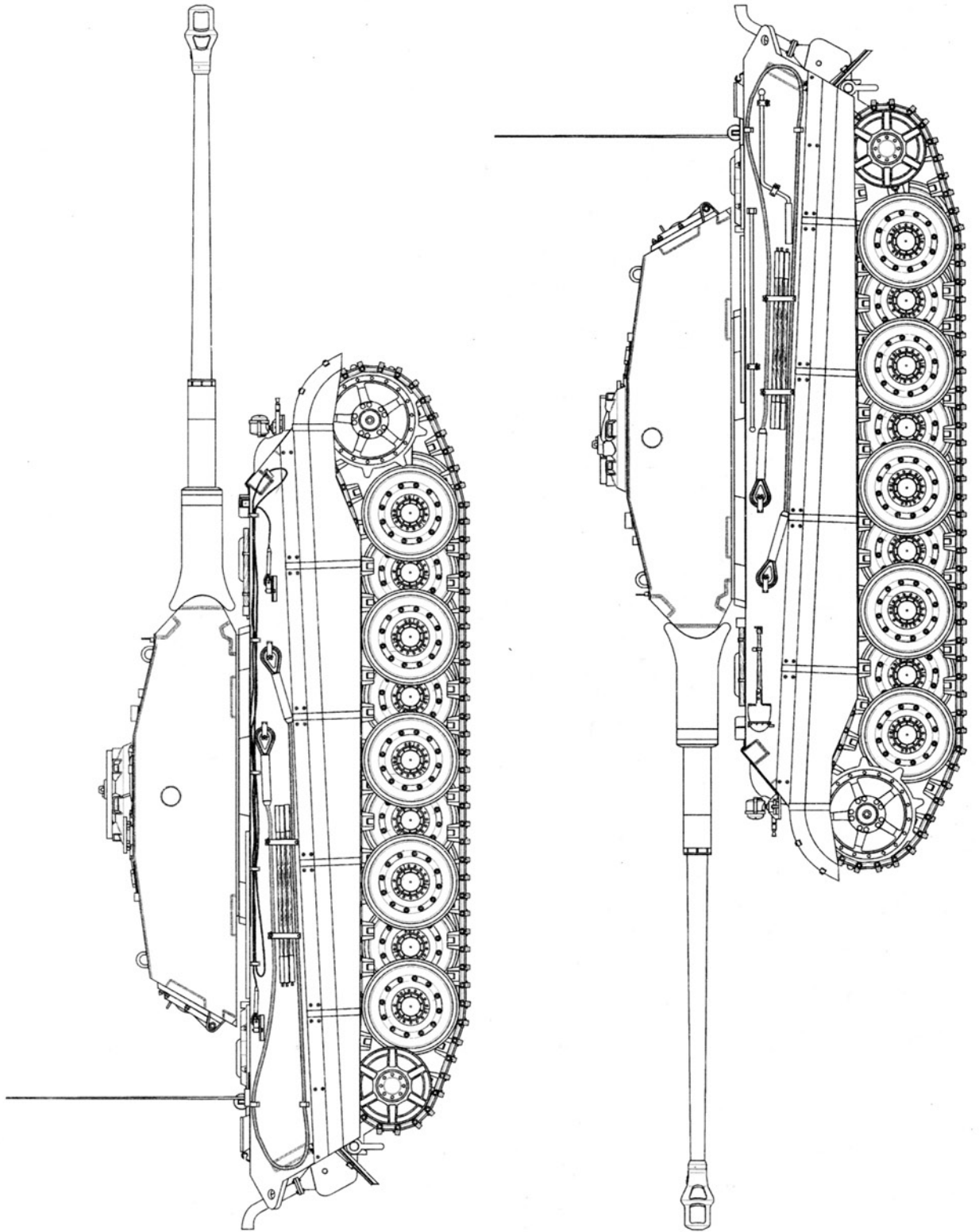
Тяжелый танк Pz. Kpfw. VI Ausf. B Tiger II с башней «типа Порше» Чертеж выполнил В. Мальгин
