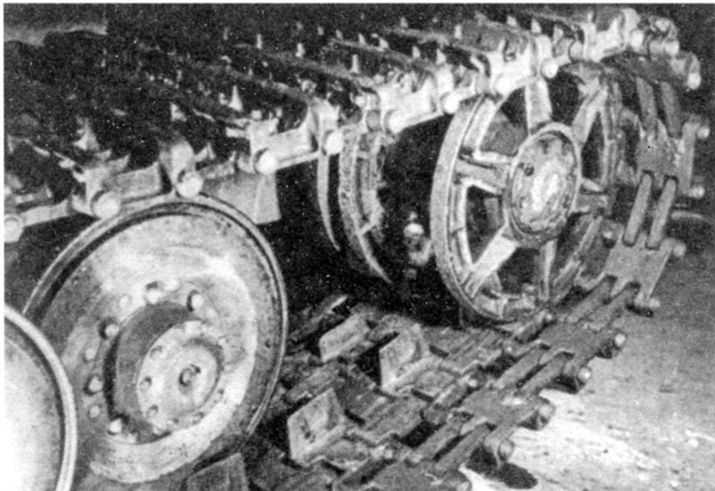
Направляющее колесо ходовой части конструкции Ф.Порше
