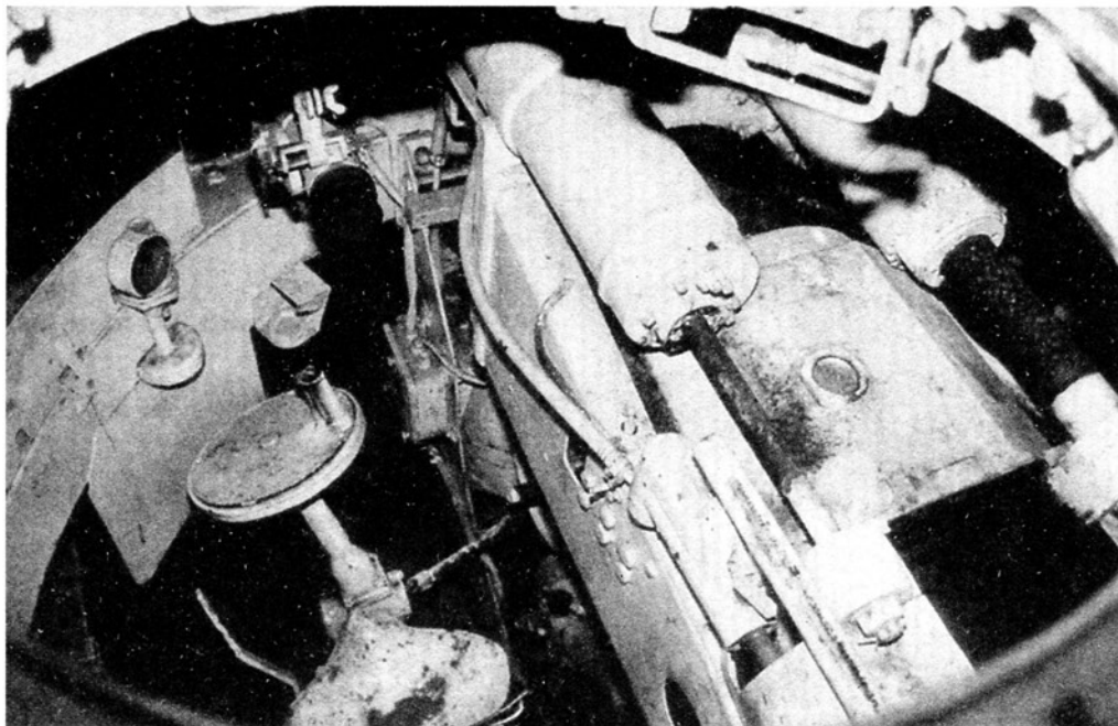
Вид в башню через люк командира. Справа — казенник пушки, слева — сиденье наводчика и маховик ручного привода механизма поворота башни
