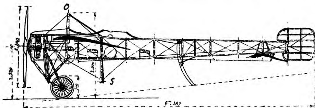
Fig. 4. Seitenriß des zweisitzigen Blériot-Eindeckers.
