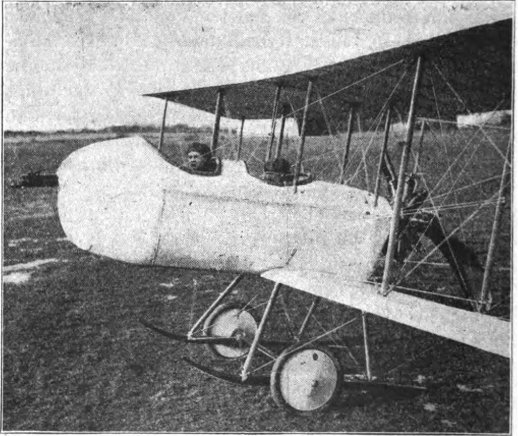
Fig. 89. Vickers-Zweidecker mit Maschinengewehr.
