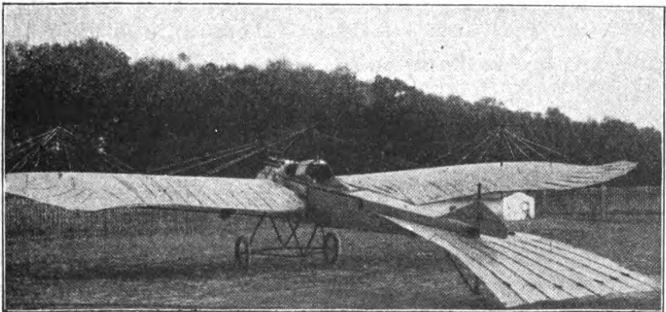
Fig. 66. D.-F.-W.-Stahltaube.
