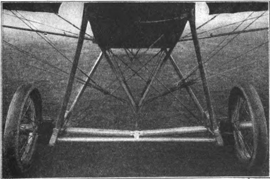
Fig. 68. Fahrgestell der Roland-Taube.
