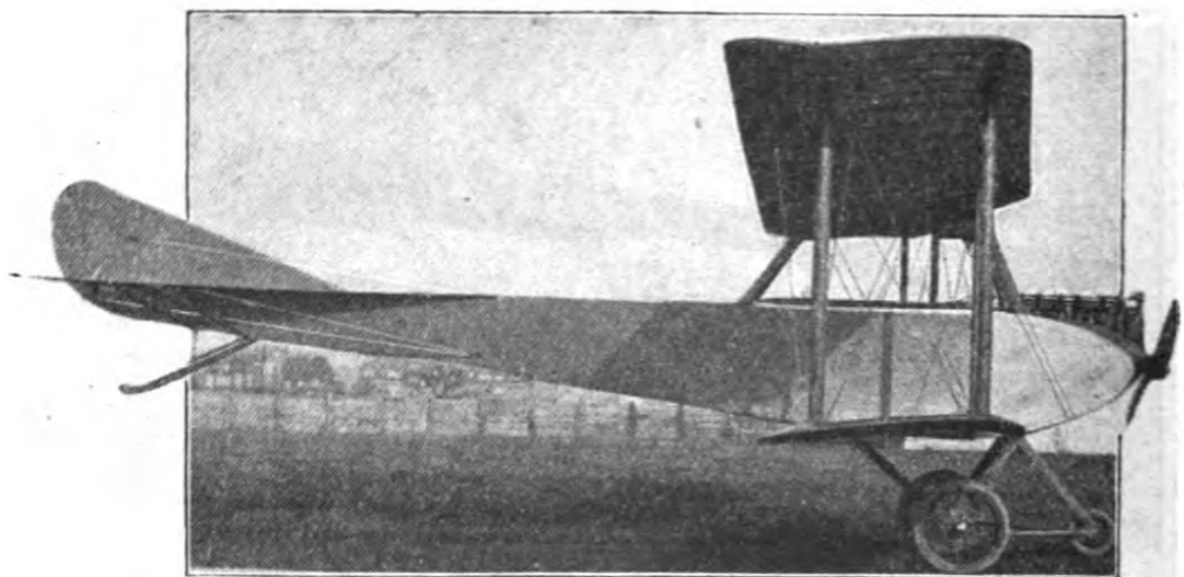
Fig. 108. Euler-Zweidecker, Militär-Typ.
