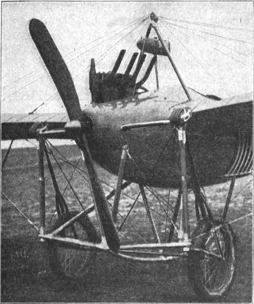
Fig. 55. Etrich-Taube, Fahrgestell.
