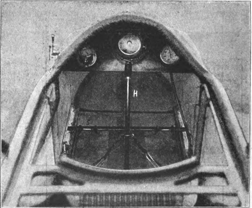
Fig. 86. Führersitz im Otto-Doppeldecker. H = Handhebel für Höhensteuer und Verwindung. S = Seitensteuerhebel.
