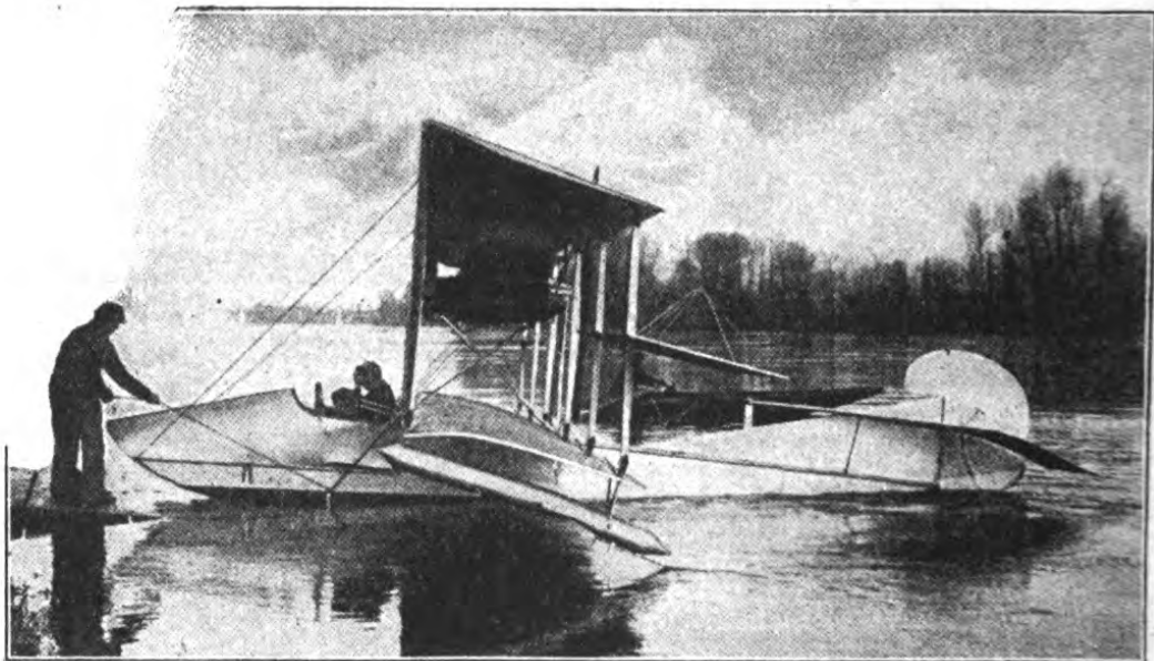
Fig. 147. Curtiss-Flugboot. Seitenansicht.
