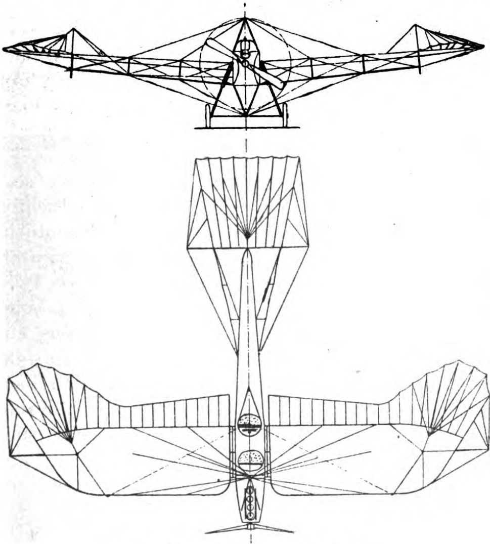
Fig. 63 und 64. Jeannin-Taube.
