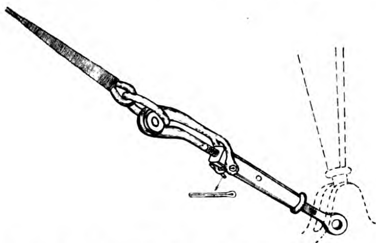
Fig. 102. Spannschloß des L.-V.-G.-Zweideckers.
