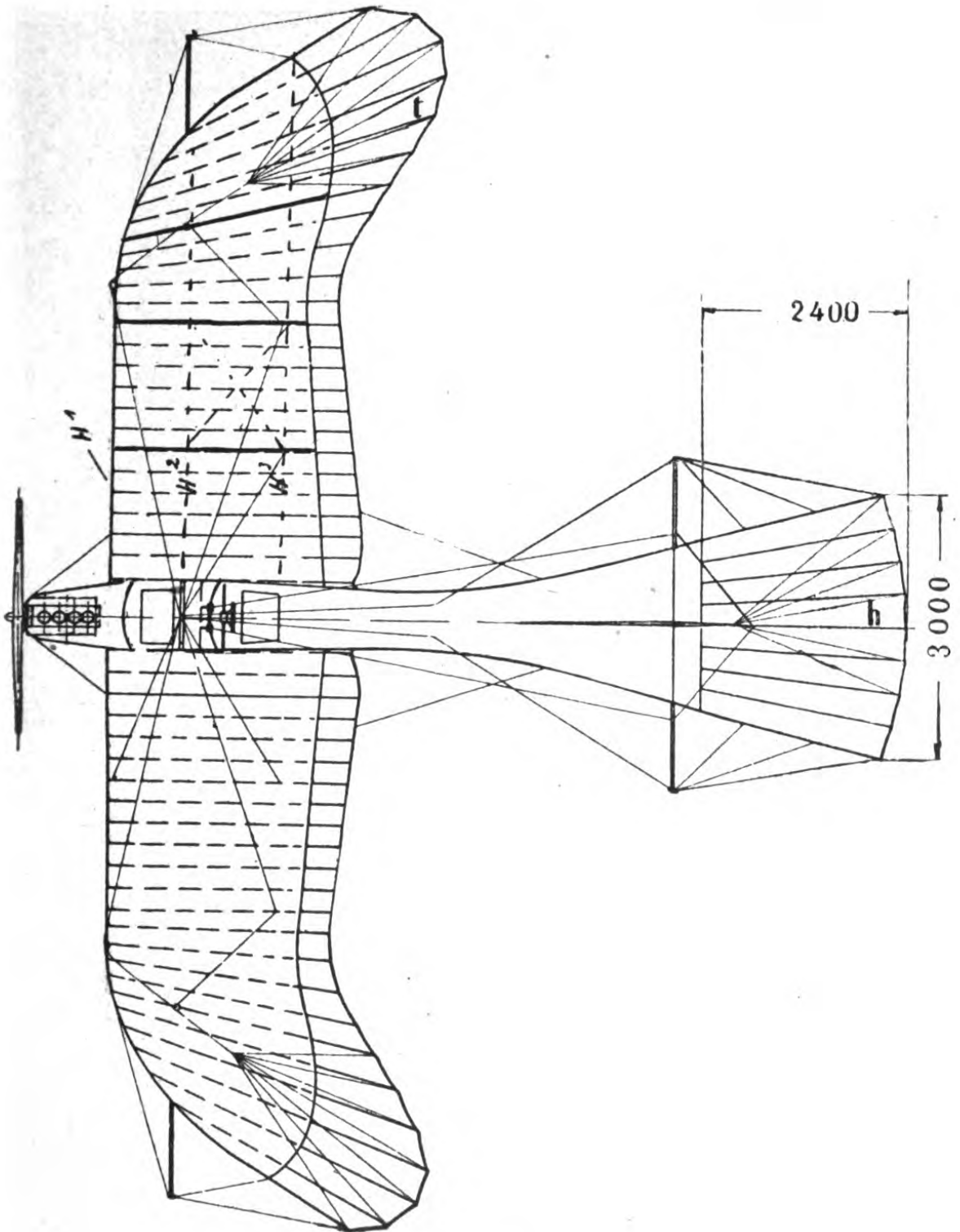
Fig. 53. Aufriß der „Taube“.
