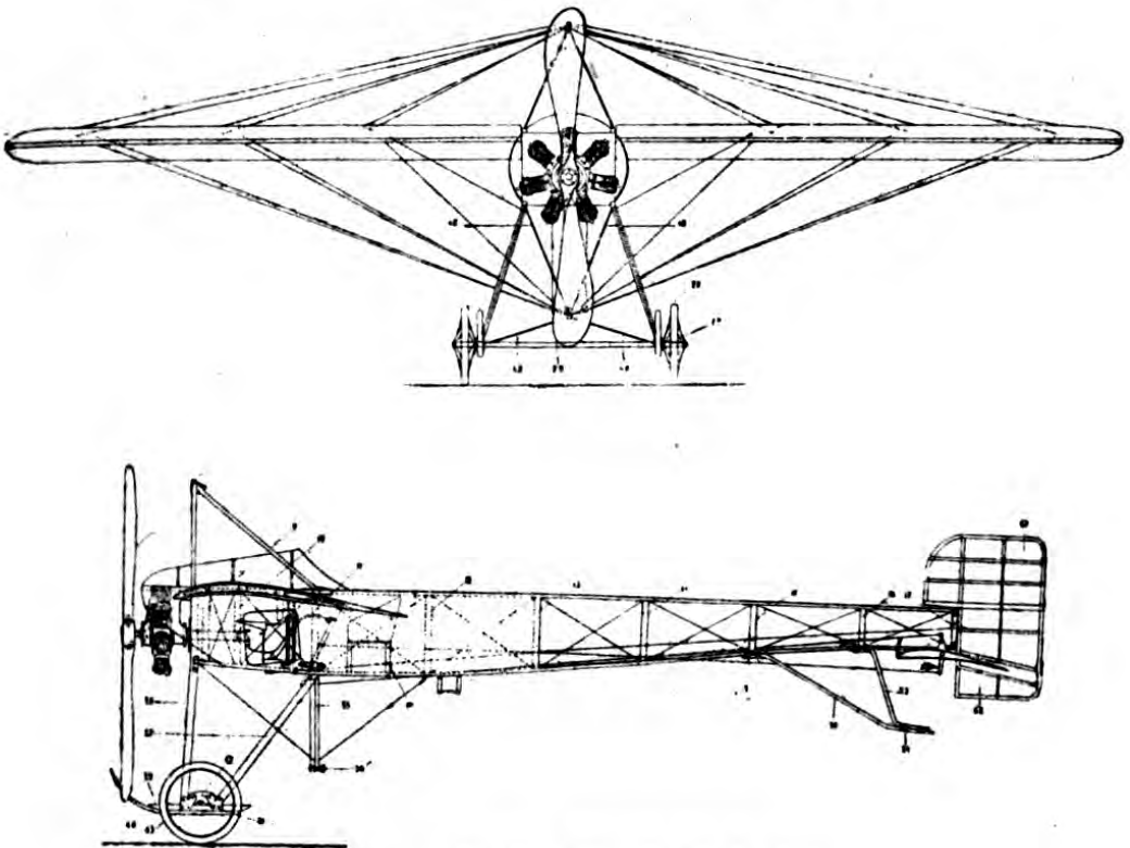
Fig. 9 und 10. Borel-Eindecker.
