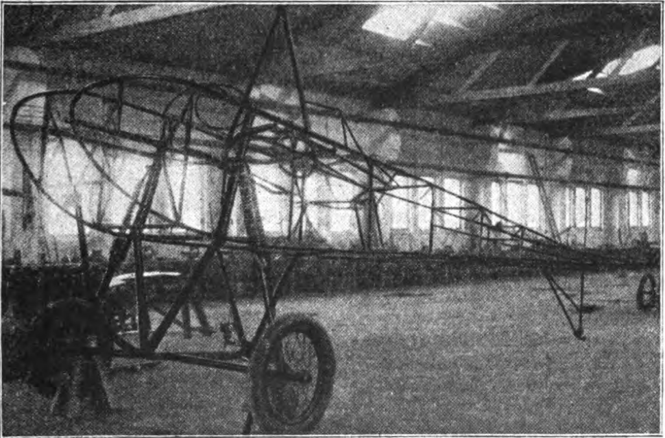
Fig. 65. Stahlrohrumpf der D.-F.-W.-Taube.
