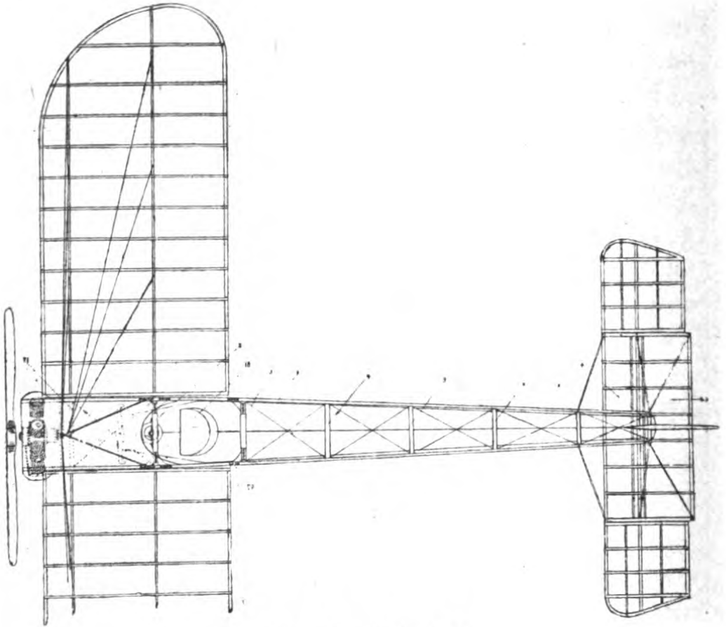
Fig. 11. Borel-Eindecker.
