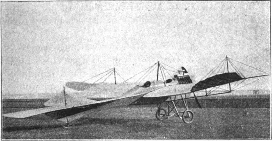
Fig. 59. Albatros-Taube, Seitenansicht.
