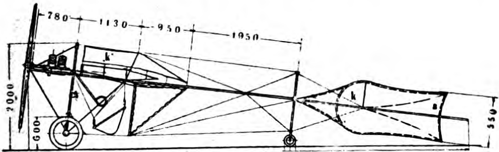
Fig. 44. Erster Grade-Eindecker. Nach: „Der Flugsport“.
