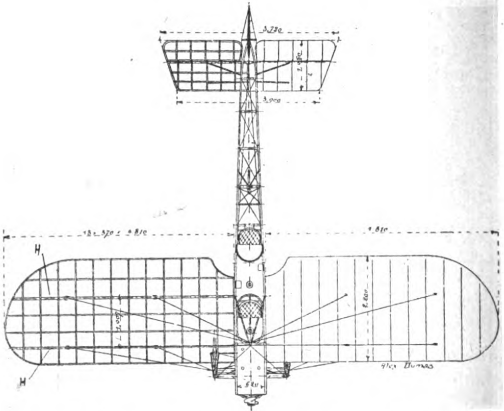
Fig. 5. Grundriß des zweisitzigen Blériot-Eindeckers.
