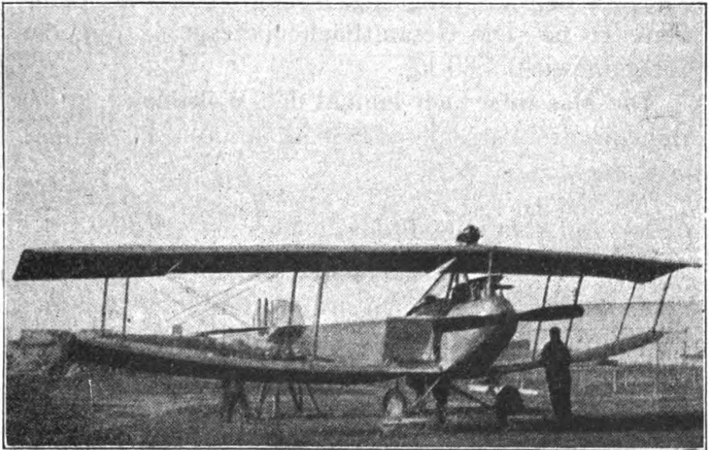
Fig. 132. Union-Pfeil-Zweidecker.
