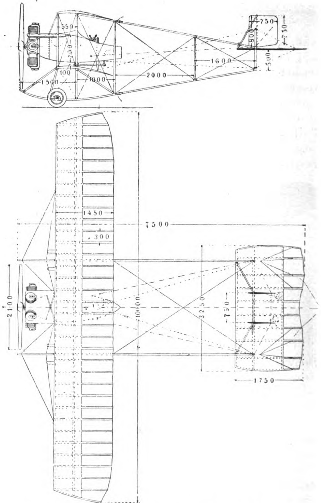
Fig. 94 und 95. Caudron-Zweidecker, Auf- und Seitenriß (Nach: „Der Flugsport“.)
