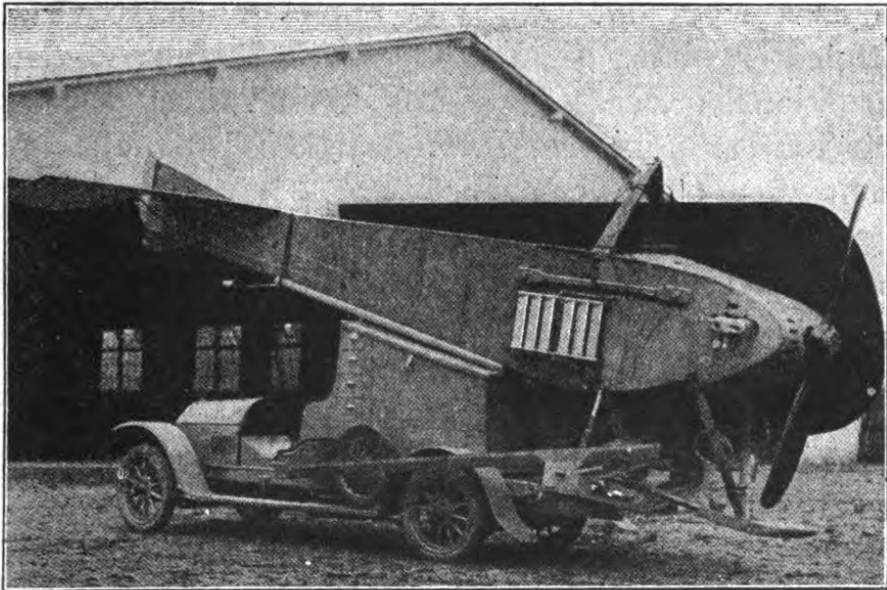
, Fig. 30. Transportwagen für den L.-V.-G.-Eindecker.
