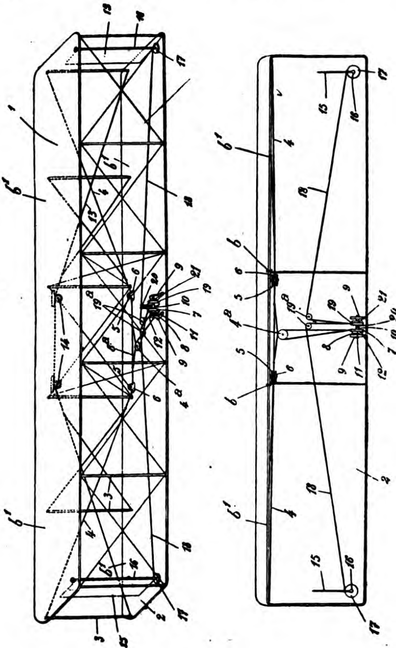
Fig. 70. Zeichnung aus der französischen Patentschrift, Drachenflieger Gebr. Wright. 1 u. 2 Tragflächen, 15 u. 16 Seitensteuerflächen, 10 u. 11 Steuerhebel mit 13 u. 18 Spannseile, 4 u. 5 Rollen zur Führung der Spannseile und zum Verwinden.
