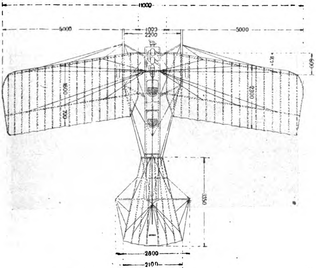
Fig. 36. Aufriß des Fokker-Eindeckers. Nach: „Der Flugsport“.
