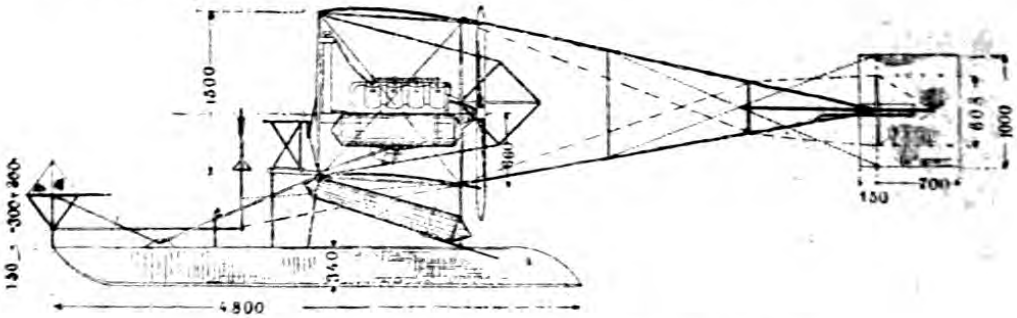
Fig. 145. Curtiss-Wasserflugzeug, alter Typ.
