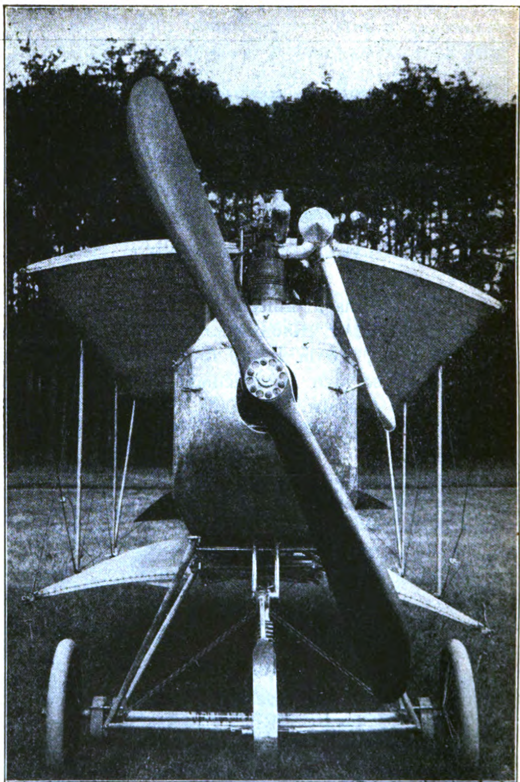
Fig. 119. Der A.-E.-G.-Zweidecker in zusammengelegtem Zustande.
