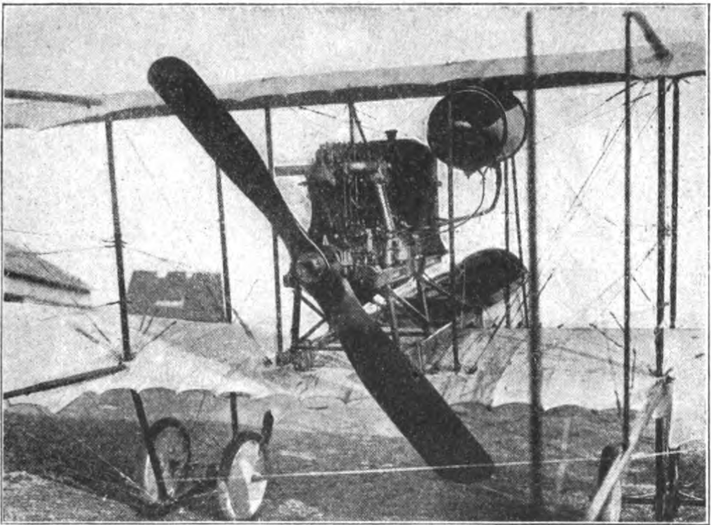
Fig. 85. Otto-Zweidecker, Rückansicht.
