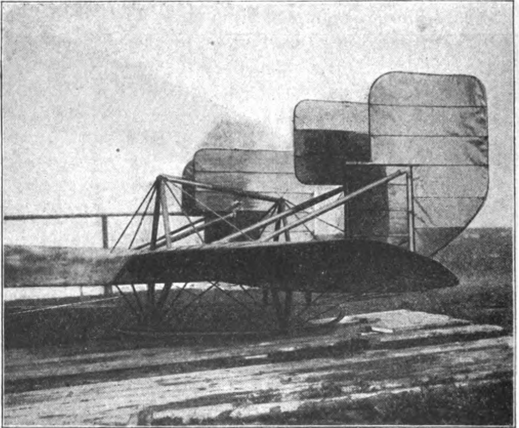
Fig. 142. Schwanz und Steuerflächen des Sikorsky-Zweideckers.
