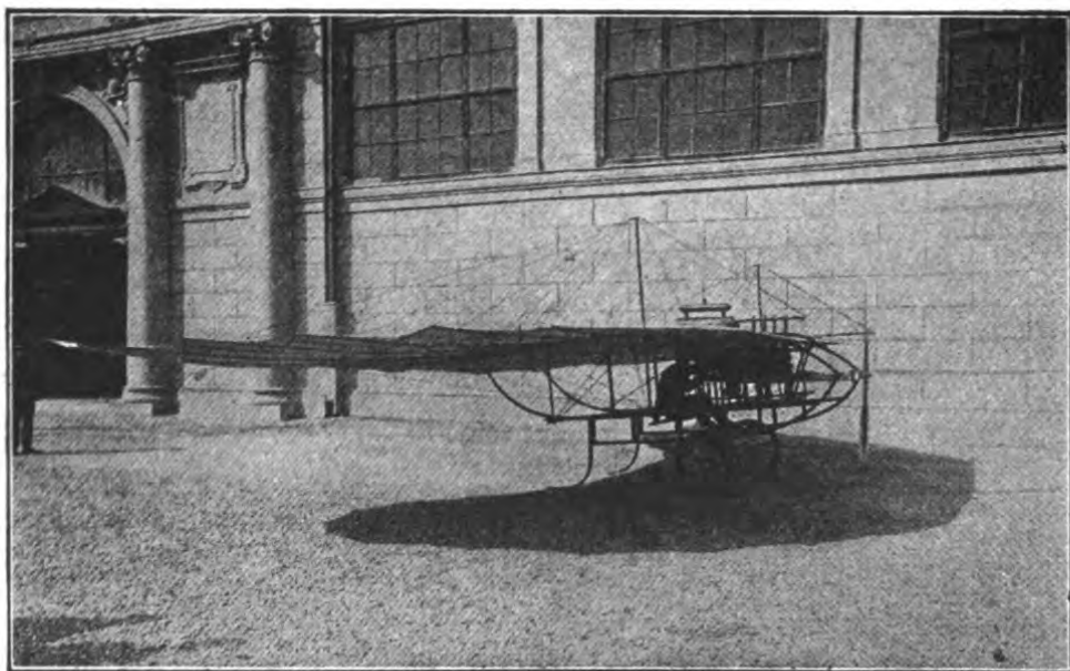
Fig. 49. Der Gleitflieger mit eingebautem Motor.
