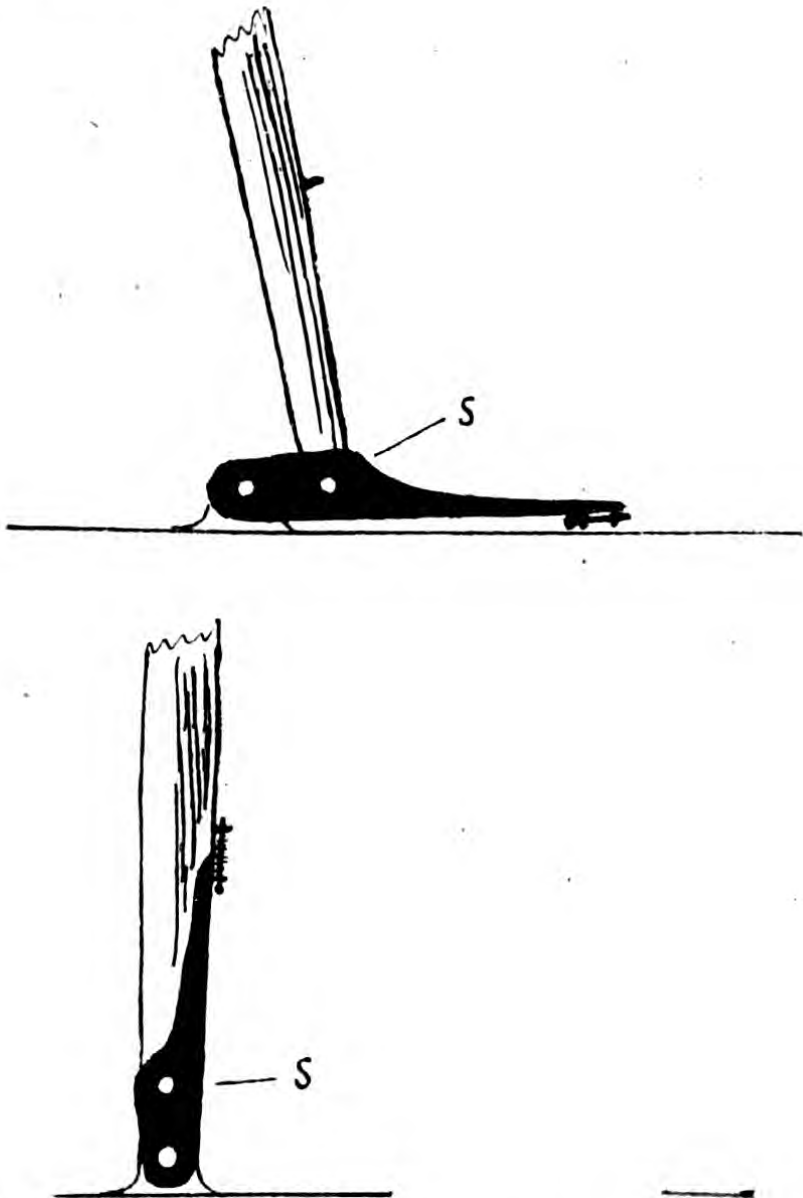
Fig. 114. Strebenverkürzung beim D.-F.-W.-Zweidecker.
