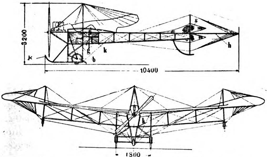
Fig. 51 und 52. Etrich-Taube. Nach: „Der Flugsport“. Die Kufe K ist heute verschwunden. k = Kühler, g = Steuersäule, b = Bremse, s = Seitensteuer, h = Höhensteuer.
