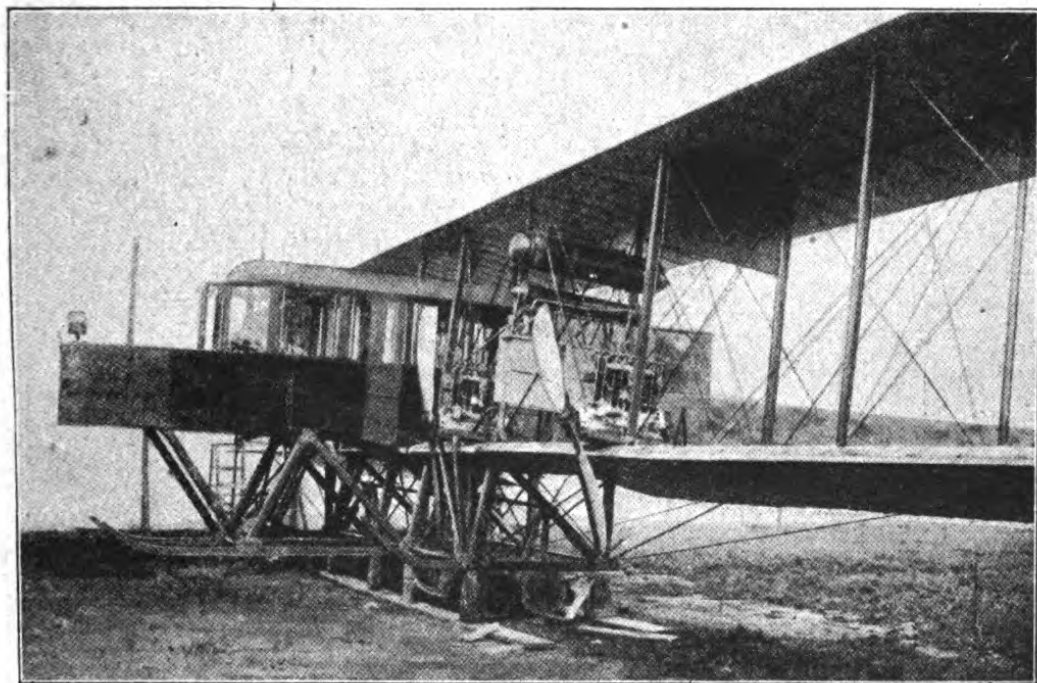
Fig. 141. Sikorsky-Zweidecker, Kabine und Motoren.
