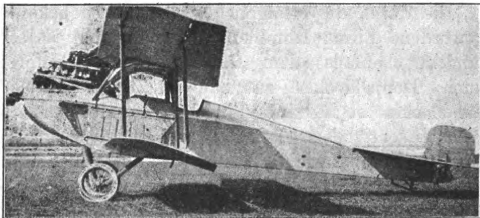
Fig. 109. Otto-Zweidecker.
