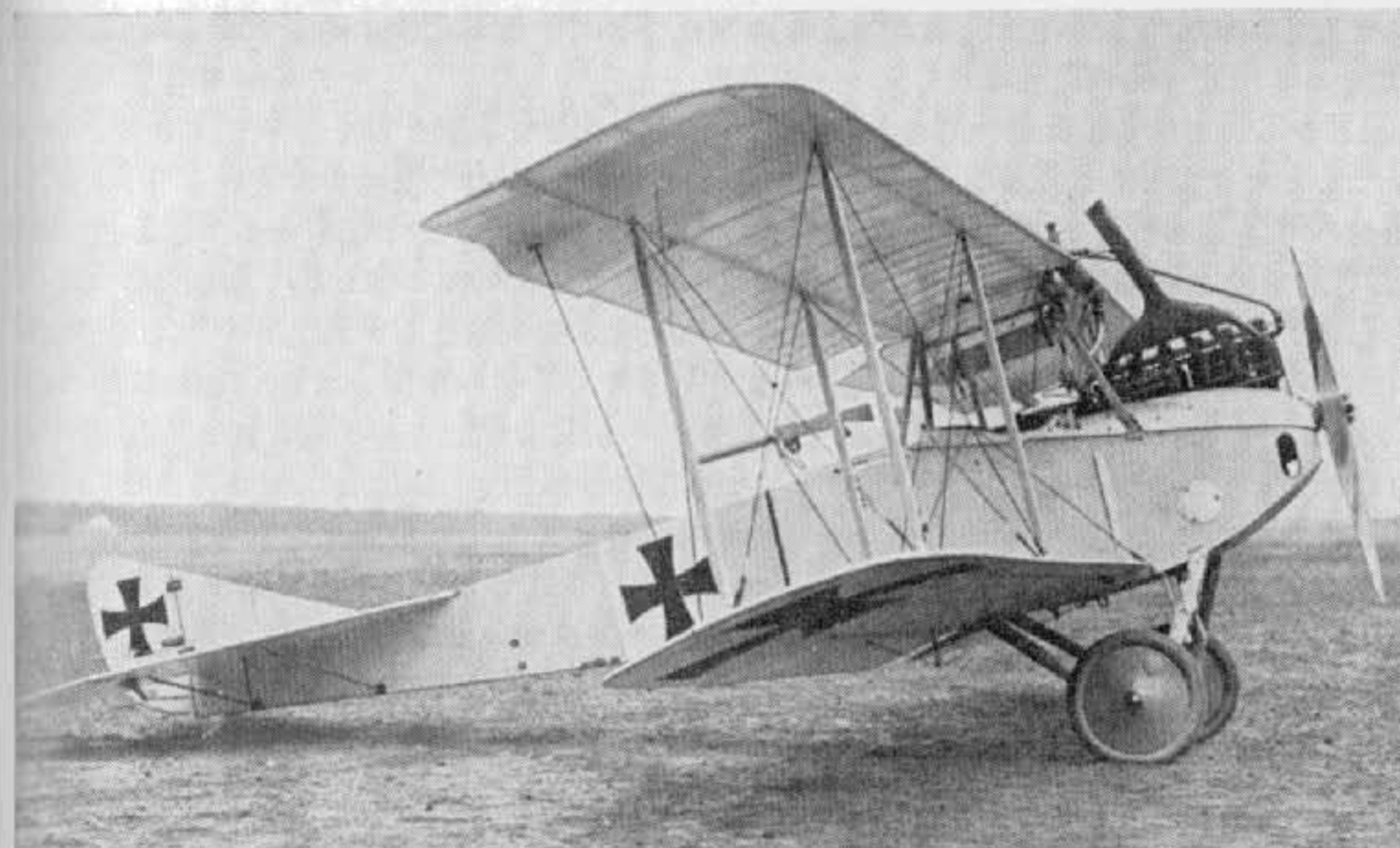
L.V.G. C II. (Photo: A. Imrie.)
