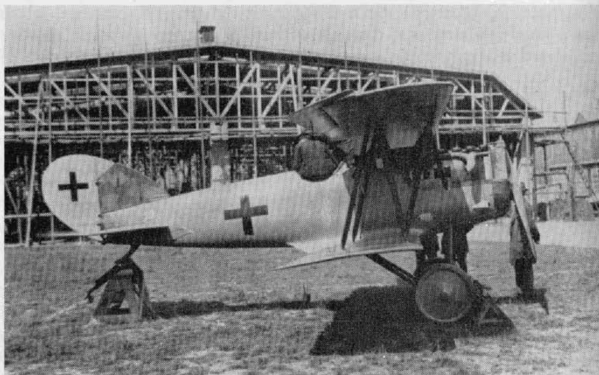
Pfalz D XII.
