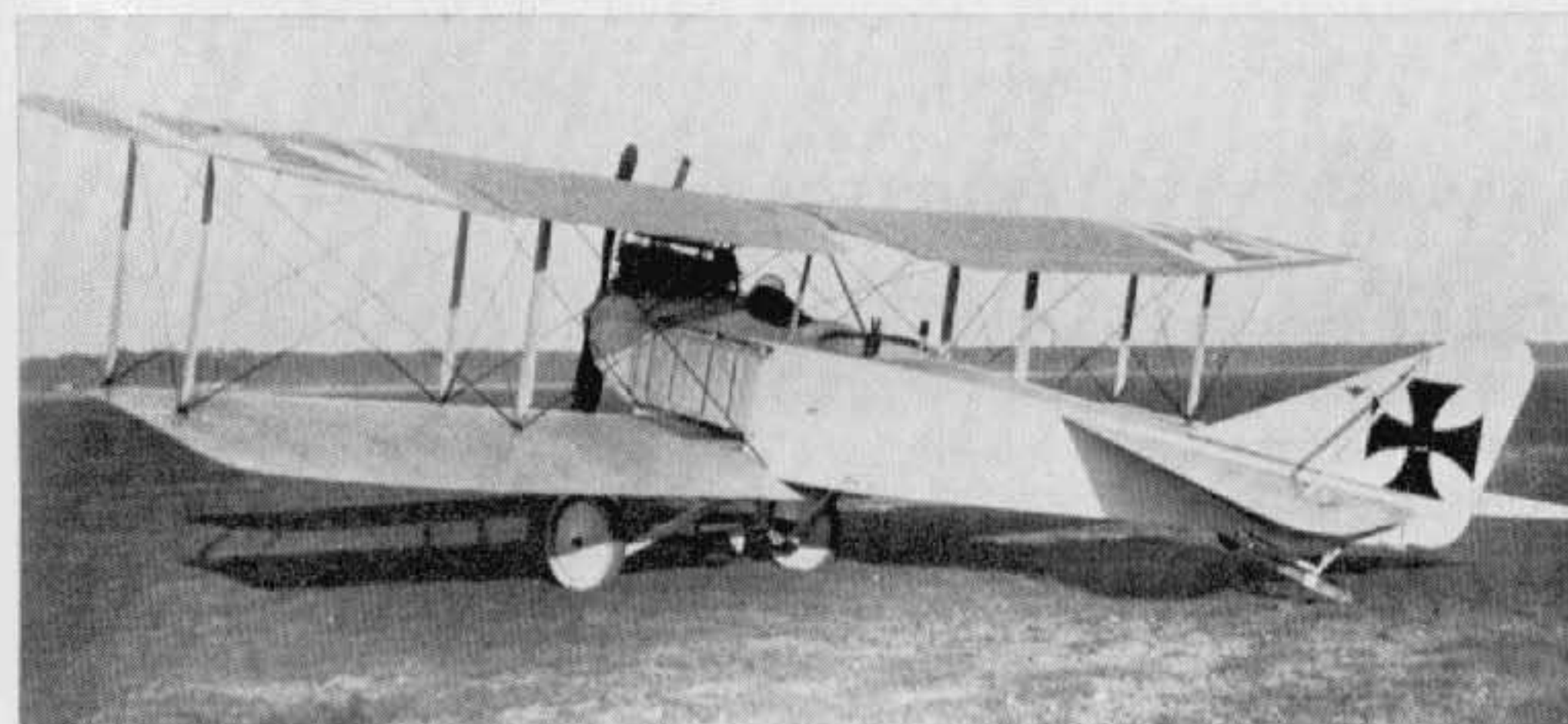
Albatros C I (160 h.p. Mercedes). (Photo: Imp. War Museum.)
