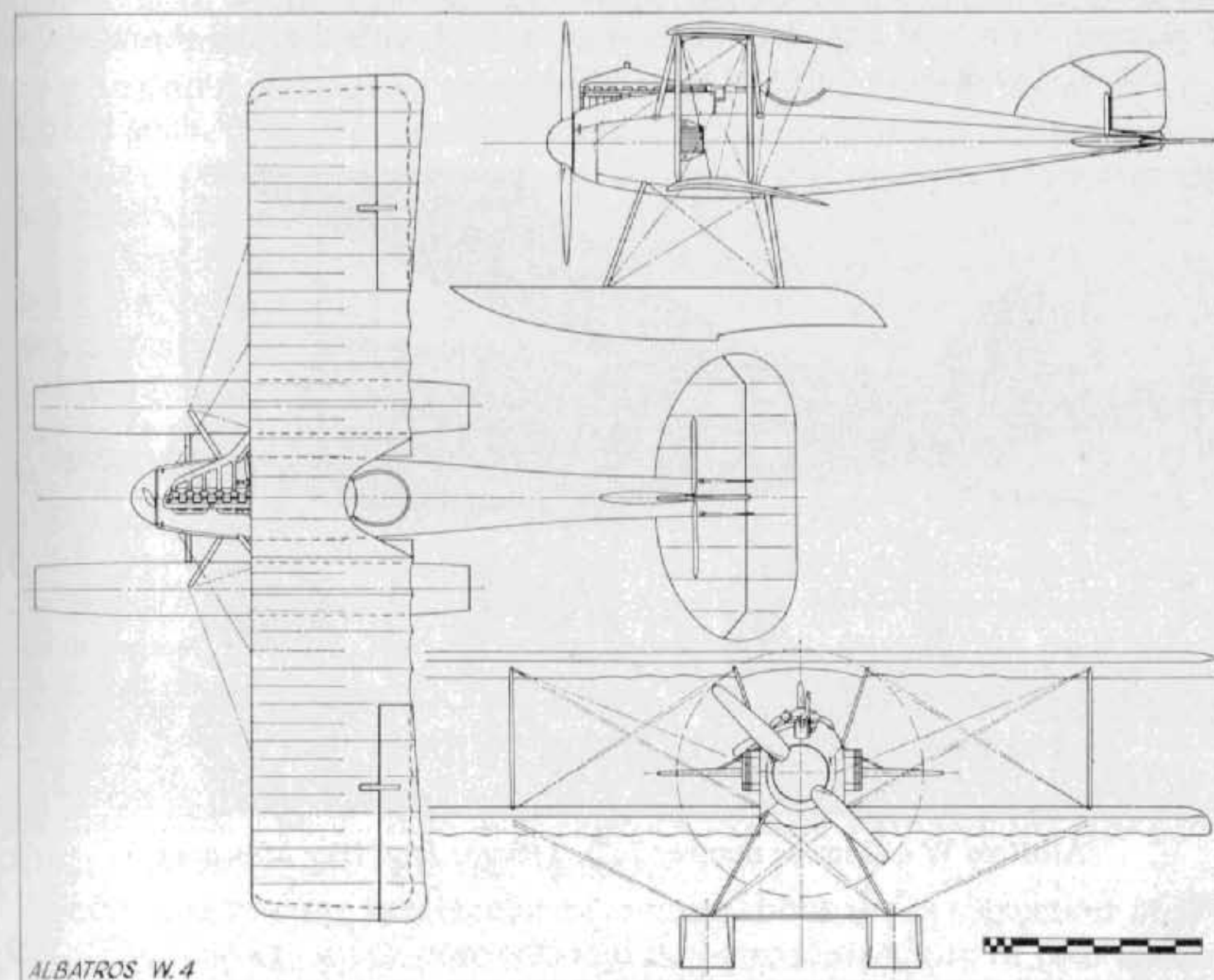
ALBATROS W.4
