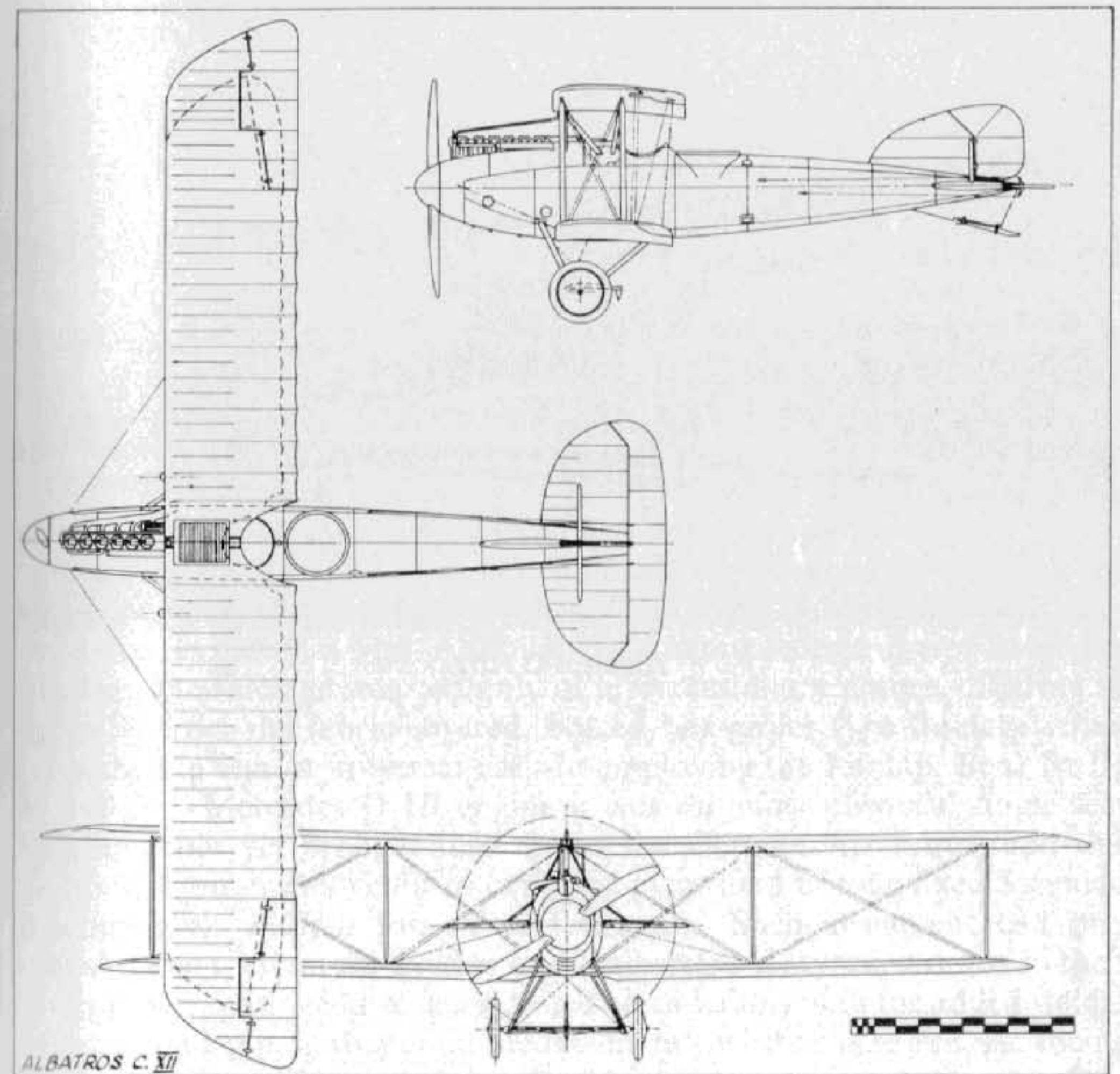
ALBATROS C. XII
