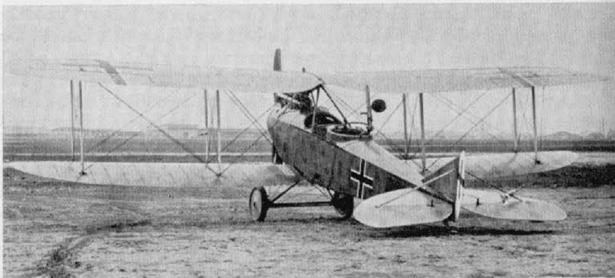
Rumpler C VII. (Photo: A. Imrie.)
