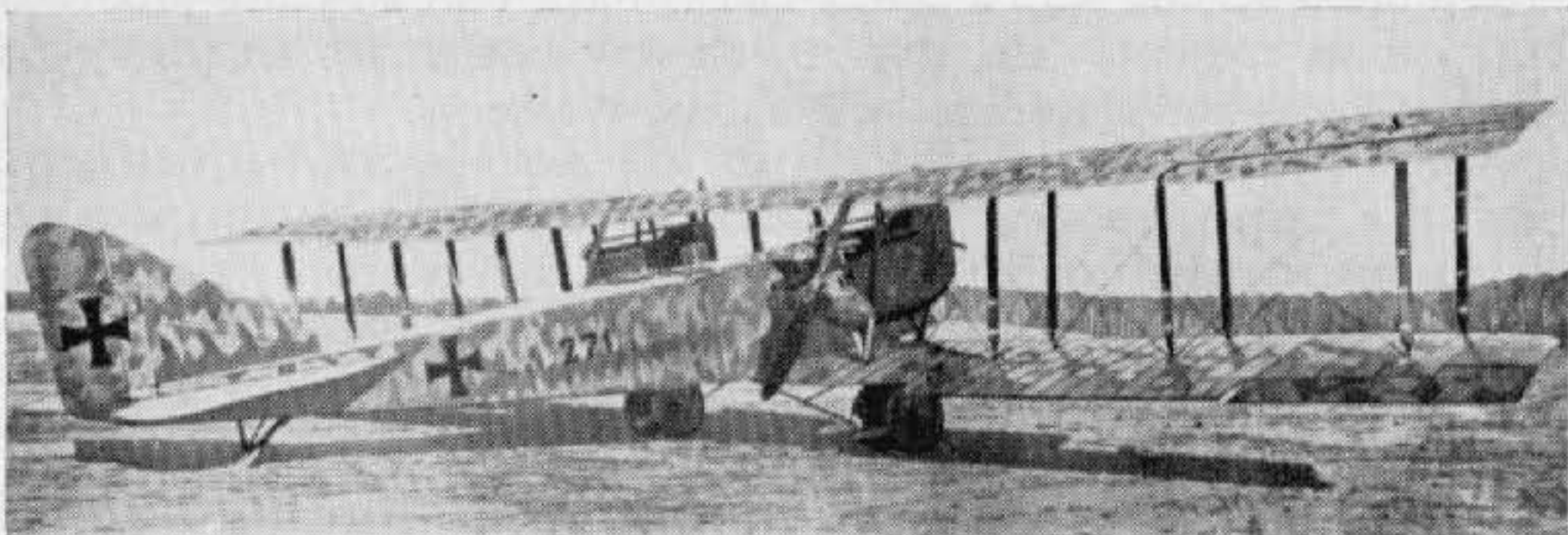
Friedrichshafen G III (serial 271/17).
