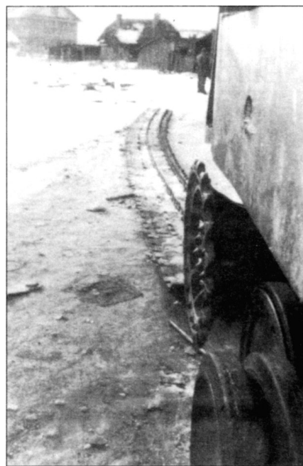
Танк «Тигр» в полевых ремонтных мастерских. В борту корпуса видна пробоина от 85-мм бронебойного снаряда.
