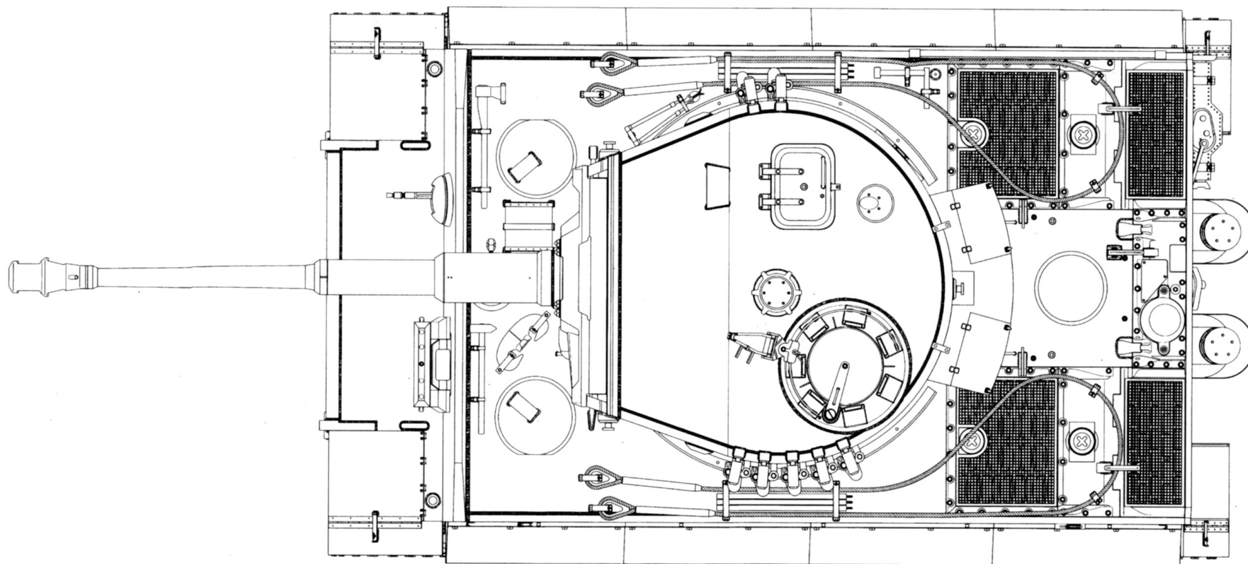
Модернизированный танк Pz.Kpfw. VI Tiger Ausf. E позднего выпуска ранней серии.
