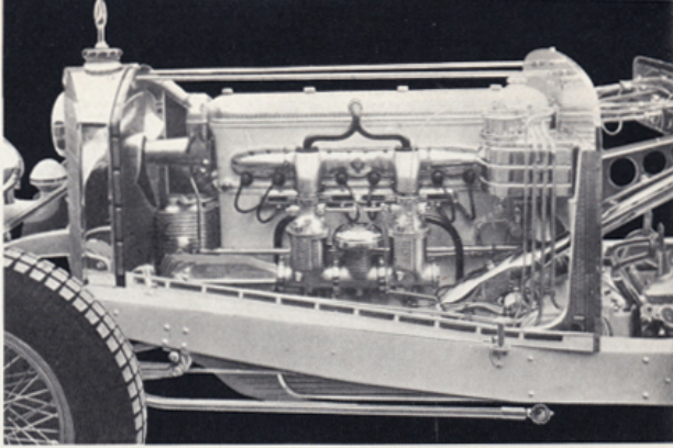
MOTOR-VERGASERSEITE
