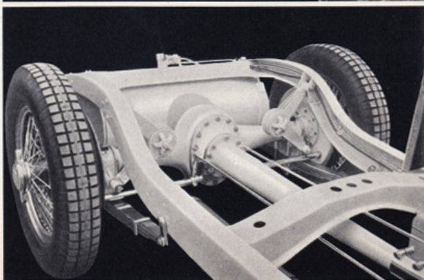
HINTERACHSBRÜCKE
