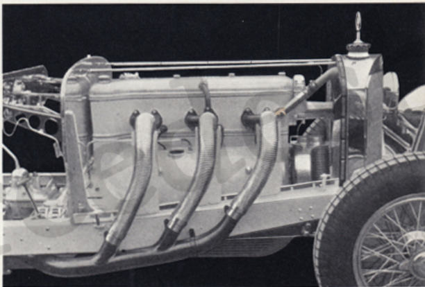
MOTOR-AUSPUFFSEITE
