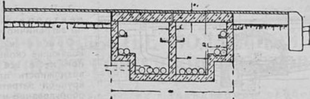
„Короб“ под тротуаром для размещения новых кабелей сильного и слабого токов
