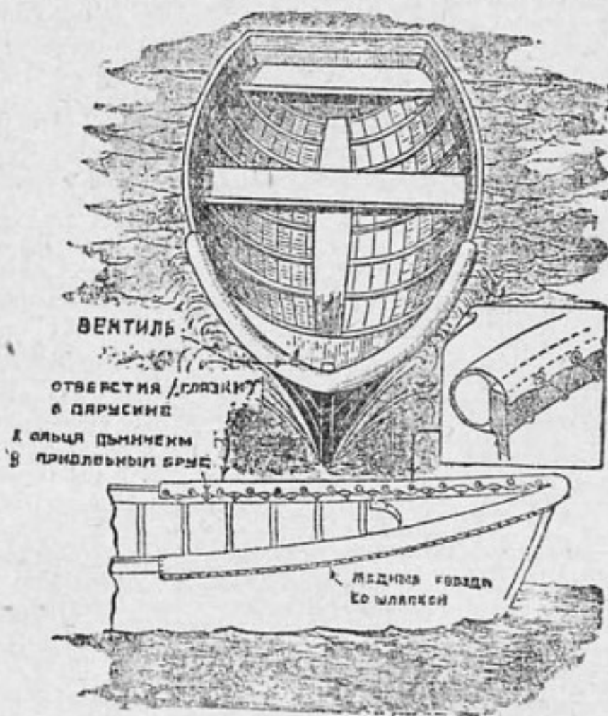
Рис. 9. Как бороться с захлестыванием носовой части
