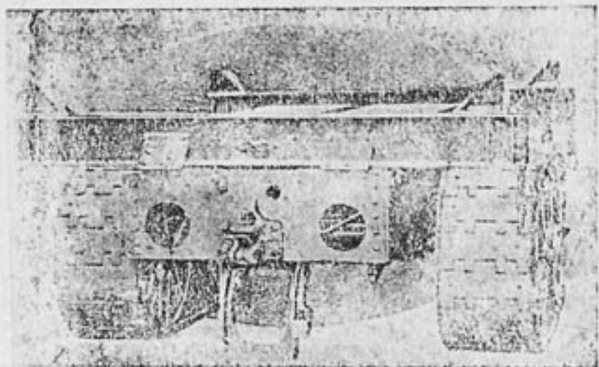
Подставки и раме Атеевской тележки, придающей ей устойчивость при погрузке. На раме виден удобный самозапирающийся прицепной крюк для сцепления тележек в поле
