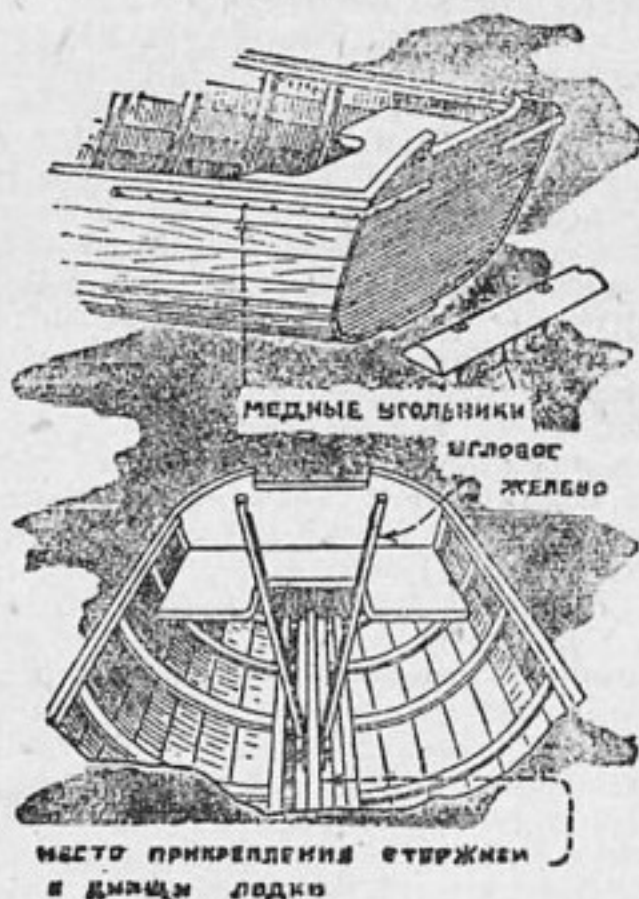
Рис. 6. Укрепление транца
