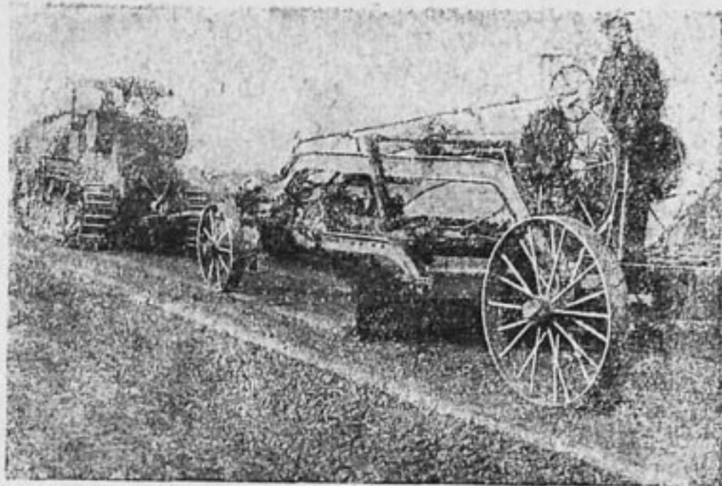
Автооструг на работе по устройству дорожного полотна
