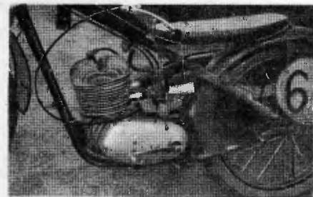
Двигатель мотоцикла одессита В. Бураčkova (третье место в классе 125 см 3 ) с трехканальной продувкой.
