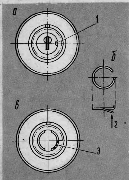
Рис. 5. Фиксация цилиндра с сувальдами в замке зажигания: а — корпус замка; б — запорная шайба; в — замок при вынудом цилиндре. 1 — вырез в цилиндре; 2 — направленные отжима уса; 3 — углубления в корпусе.
