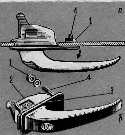
Рис. 3. Ручка двери автомобиля ЗАЗ-96Б: а — крепление к наружной панели; б — извлечение цилиндра: 1 — гайка; 2 — окно; 3 — винт; 4 — шпилька. Стрелкой показано направление, в котором надо извлекать цилиндр.
