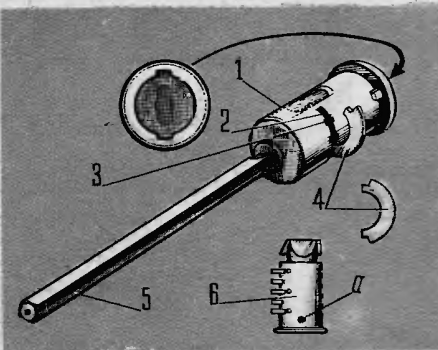
Рис. 2. Наружный выключатель замка двери у «Победы»: 1 — корпус; 2 — прорез; 3 — фиксирующие заборны; 4 — стопорная шайба; 5 — стержень; 6 — цилиндр с сувальдами; а — место для отверстия под штифт.
