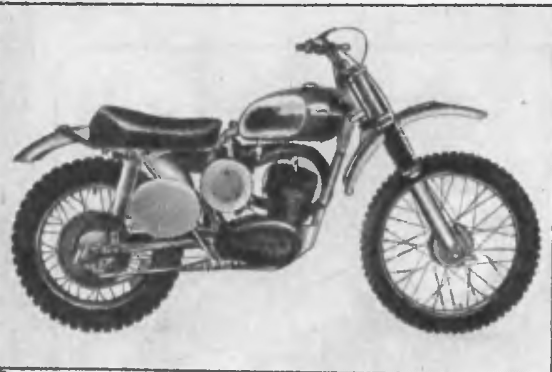
Мотоцикл «Хускварна» с двигателем класса 250 см 3 (69,5×64,5 мм, 245 см 3 ) мощностью 27 л. с. при 6500 об/мин (серийный образец). Вес 95 кг.
