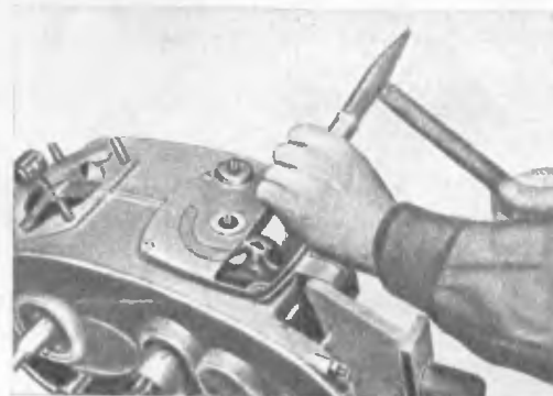
4. Регулировка пружины возврата.
