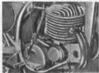
Двигатель мотоцикла «Гривс» класса 250 см 3 (70×64 мм, 248 см 3 ), развивающий мощность 27 л. с. при 5600 об/мин. Отличительная особенность — широкий рабочий диапазон оборотов — 2000 об/мин.
