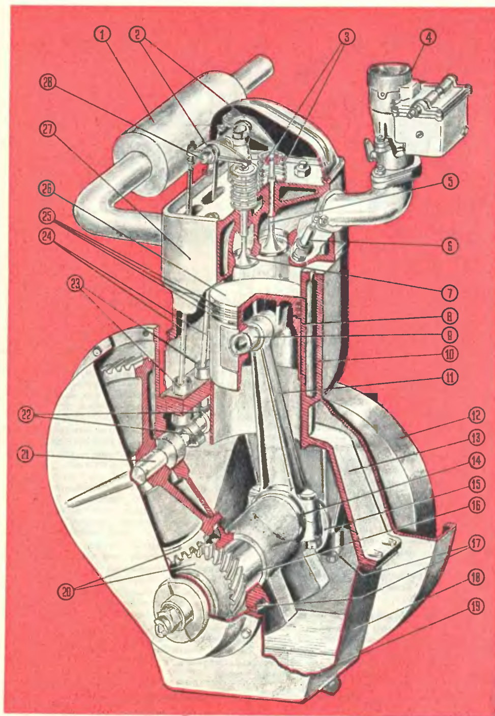
1. Карбюраторный двигатель внутреннего сгорания: 1 — глушитель; 2 — коромысла; 3 — клапанные пружины; 4 — карбюратор; 5 — впускной клапан; 6 — свеча зажигания; 7 — выпускной клапан; 8 — цилиндр; 9 — поршневой палец; 10 — водяная рубашка; 11 — шатун; 12 — маховик; 13 — картер; 14 — коленчатый вал; 15 — щека коленчатого вала; 16 — коренная шейка коленчатого вала; 17 — коренные подшипники; 18 — поддон; 19 — запас масла; 20 — распределительные штанги; 21 — распределительный вал; 22 — нулачки; 23 — толкатели; 24 — клапанные коромысла.
