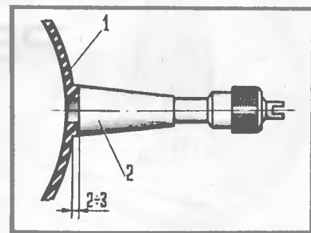
Рис. 1: 1 — камера; 2 — удаленная часть вентиля.
