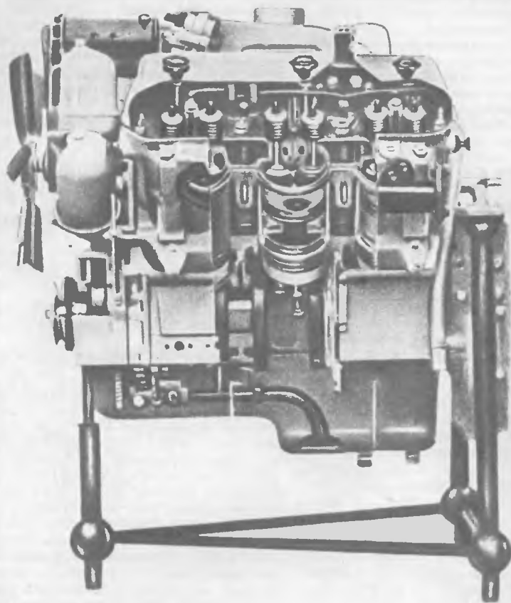
4. Общий вид учебного шестцилиндрового дизеля ЯМЗ-236 (в разрезе).
