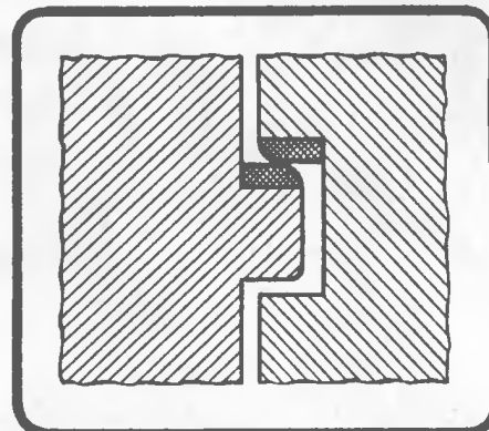
2. Закругление кромок кулачков и пазов (сечение).
