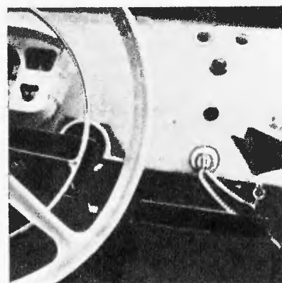
Рис. 12. Конструкция отключателя: 1 — изоляционная ая пластина; 2 — медная или латунная разрезная пластина; 3 — виит подвода «минусового» провода; 4 — панель корпуса автомобиля; 5 и 6 — болты крепления; 7 — штифт; 8 — «минусовый» провод; 9 — заклепки.
