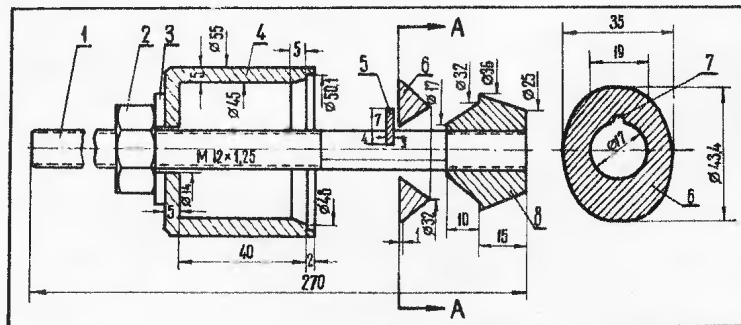
Рис. 10. Съемиинк для втулок рыча- гов передней под- вески: 1 — ходовой винт; 2 — гайка; 3 — шайба; 4 — упорный колпак; 5 — штифт; 6 — экстрактор; 7 — выемка для штиф- та; 8 — гайка эк- страктора.
