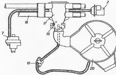
Рис. 3. Система управления подачи топлива.
