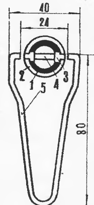
Демонтаж рычага переключения передач: 1 — резиновая втулка; 2 — отстой вала; 3 — цапфа; 4 — пружина; 5 — съемник.
