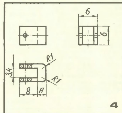
Рис. 4. Подкладка.
