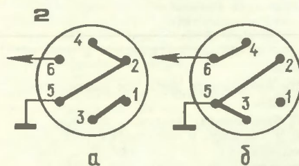
Рис. 2. Коммутация цепей в тумблере: а — положение для пуска двигателя (обмотки освещения подключены к обмоткам зажигания); б — положение после пуска двигателя.
