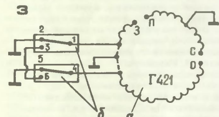
Рис. 3. Схема подключения микропереключателей МП-1: а — генератор; б — микропереключатель (положение после пуска двигателя); 3 — обмотка зажигания; О — вывод обмоток освещения; С — вывод обмотки стоп-сигнала; П — вывод обмотки указателей поворота.
