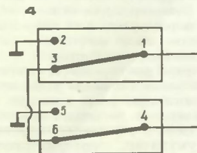
Рис. 4. Коммутация цепей в микропереключателях при пуске двигателя.
