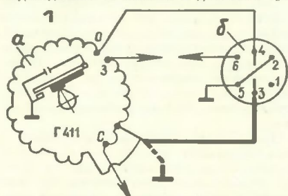
Рис. 1. Схема подключения тумблера ТП1-2: а — генератор; б — тумблер; О — вывод обмоток освещения; 3 — вывод обмоток зажигания; С — вывод обмотки стоп-сигнала. Пунктиром показано прежнее соединение обмоток с «массой», толстой линией — новое соединение.
